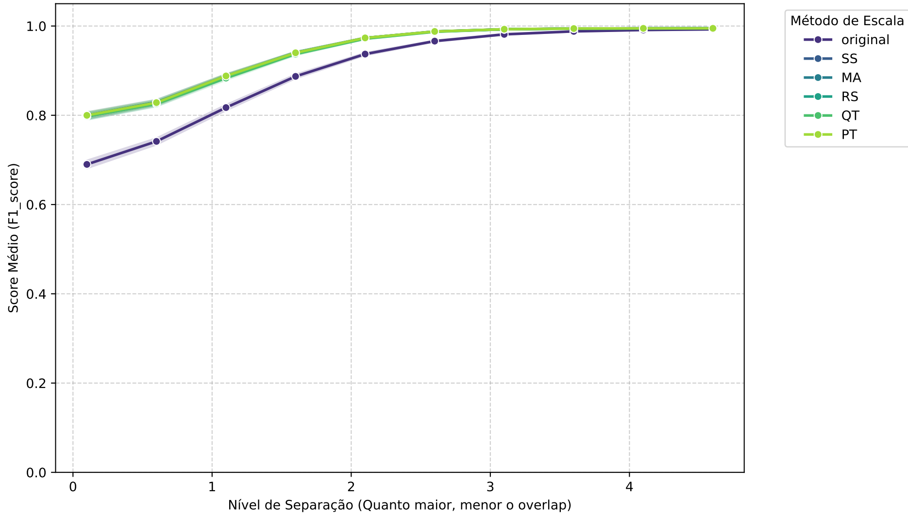
Média Geral: SVM_rbf - F1_SCORE vs Separação
