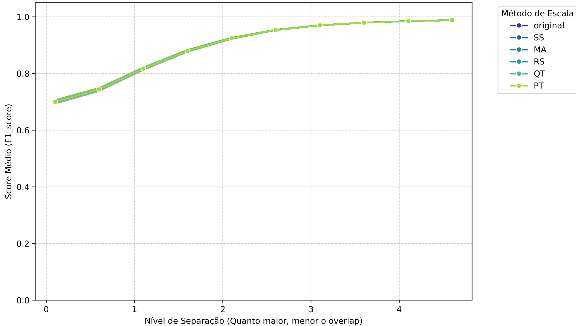
Média Geral: XGBoost - F1_SCORE vs Separação
