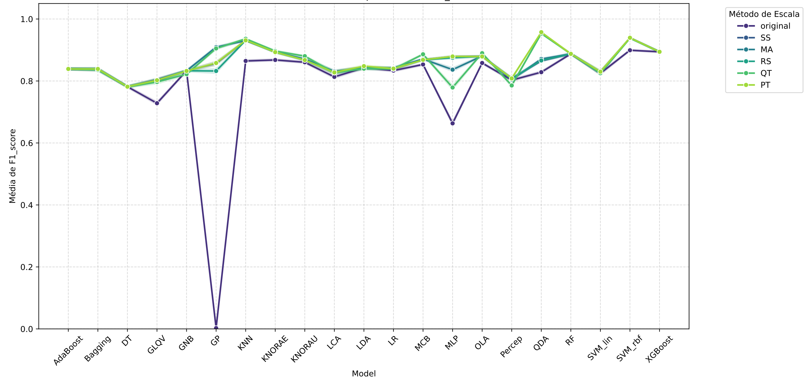
Média Global (Tendência por Modelo) - F1_SCORE
