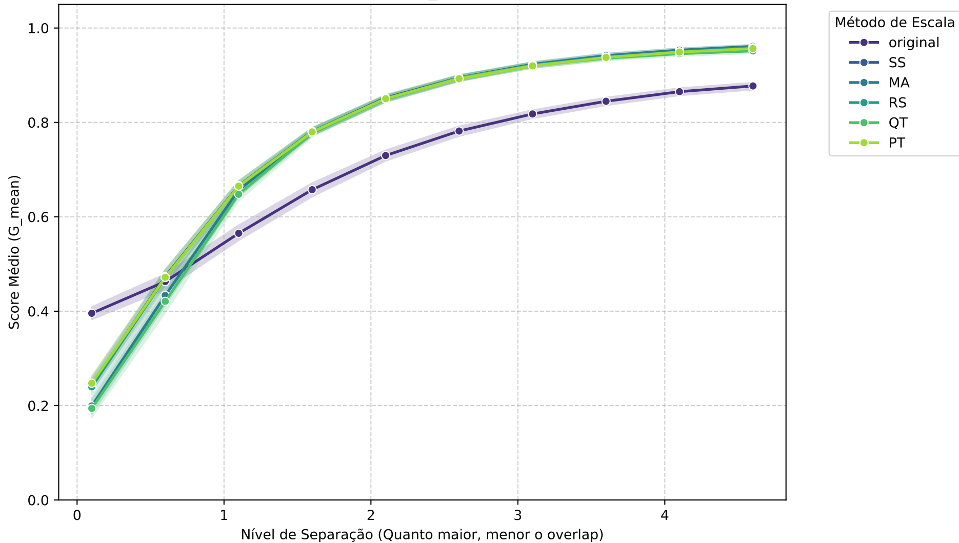
Média Geral: GLQV - G_MEAN vs Separação
