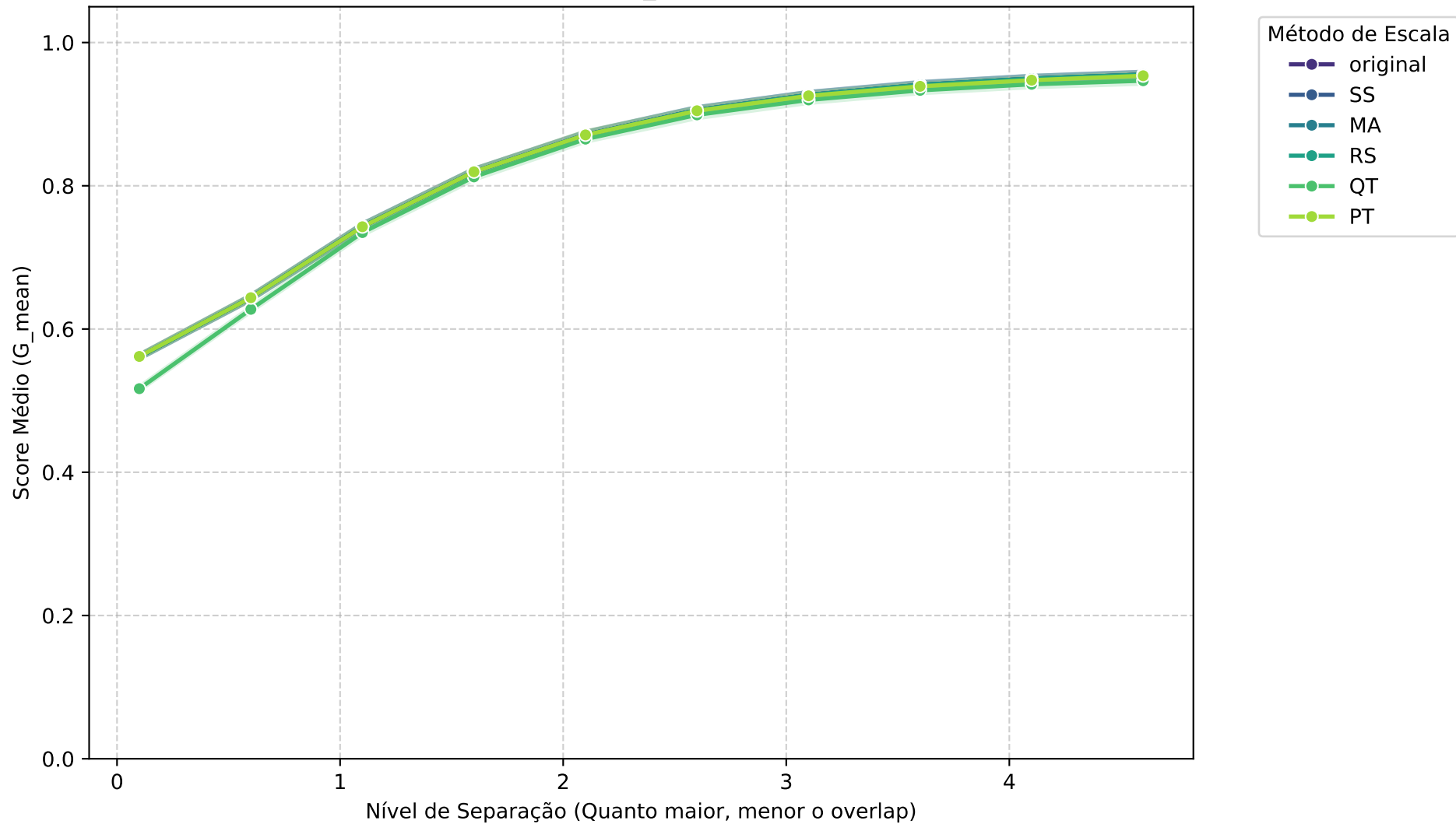
Média Geral: GNB - G_MEAN vs Separação
