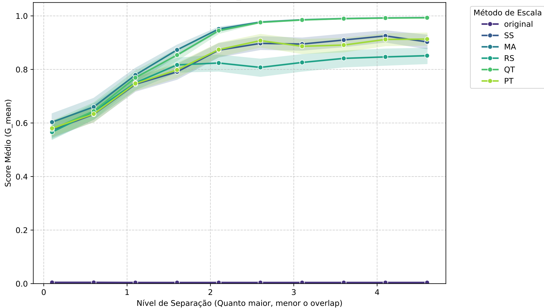
Média Geral: GP - G_MEAN vs Separação
