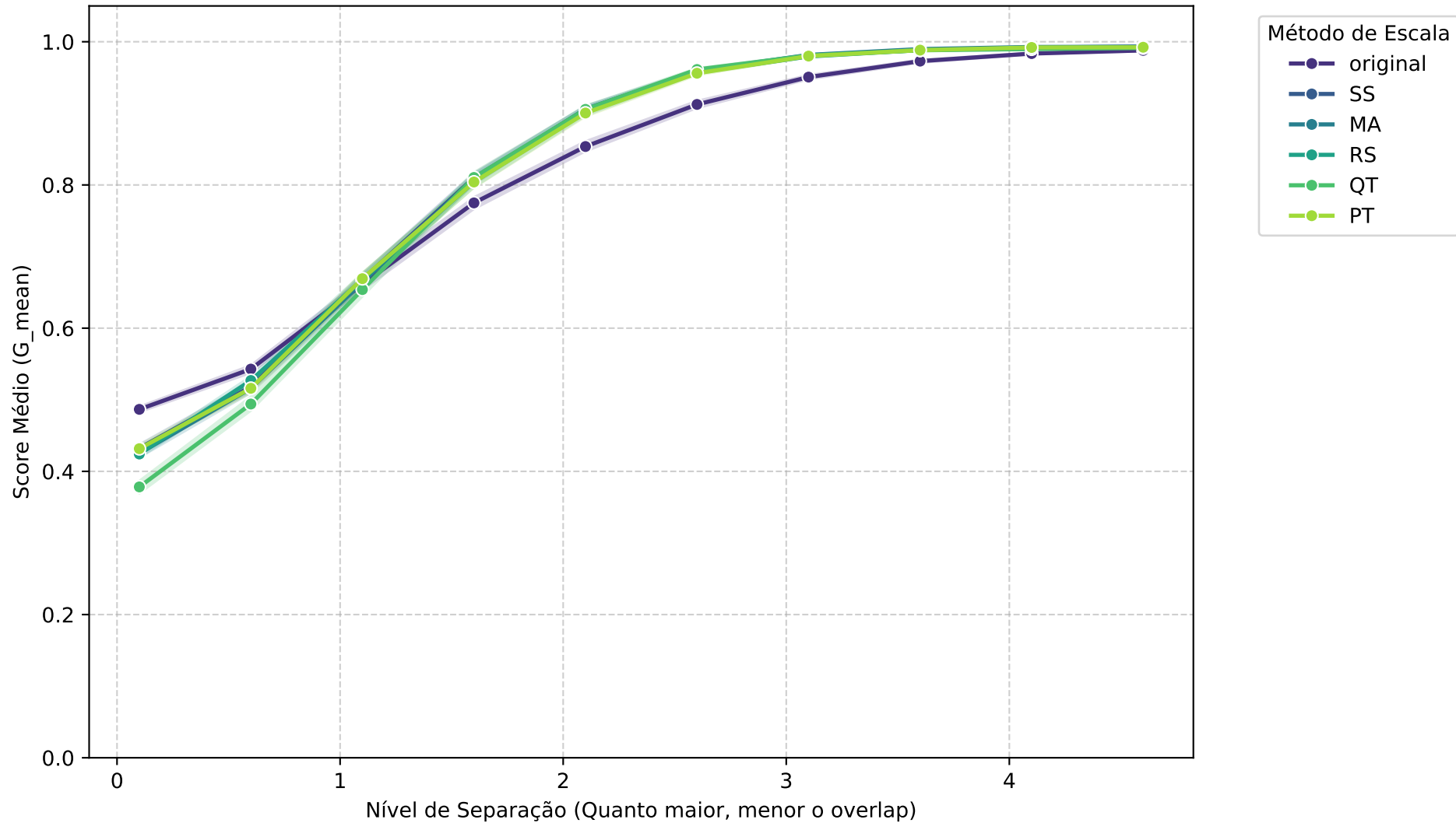
Média Geral: LCA - G_MEAN vs Separação
