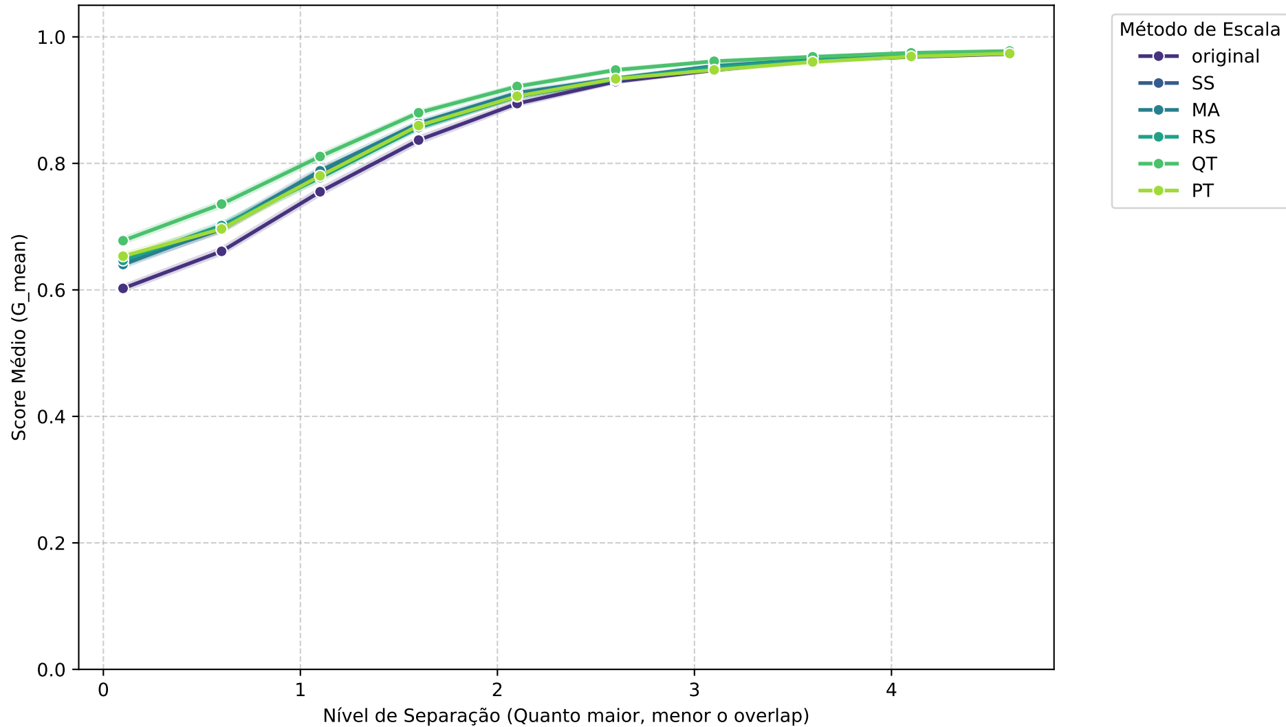
Média Geral: MCB - G_MEAN vs Separação
