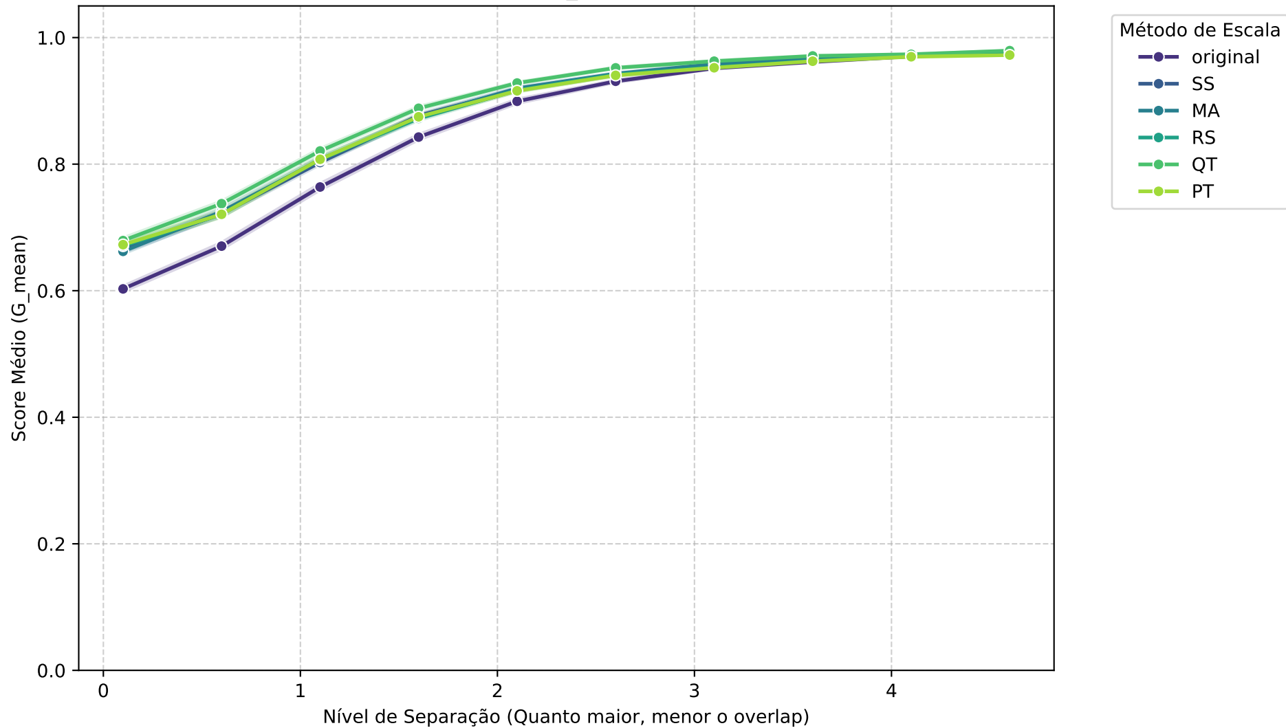
Média Geral: OLA - G_MEAN vs Separação
