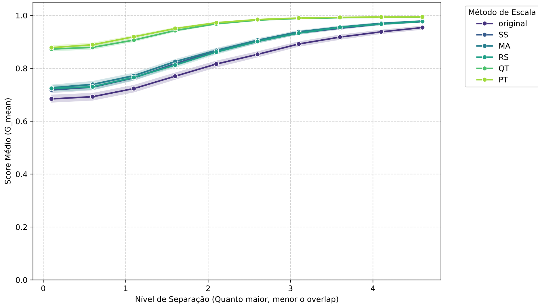
Média Geral: QDA - G_MEAN vs Separação
