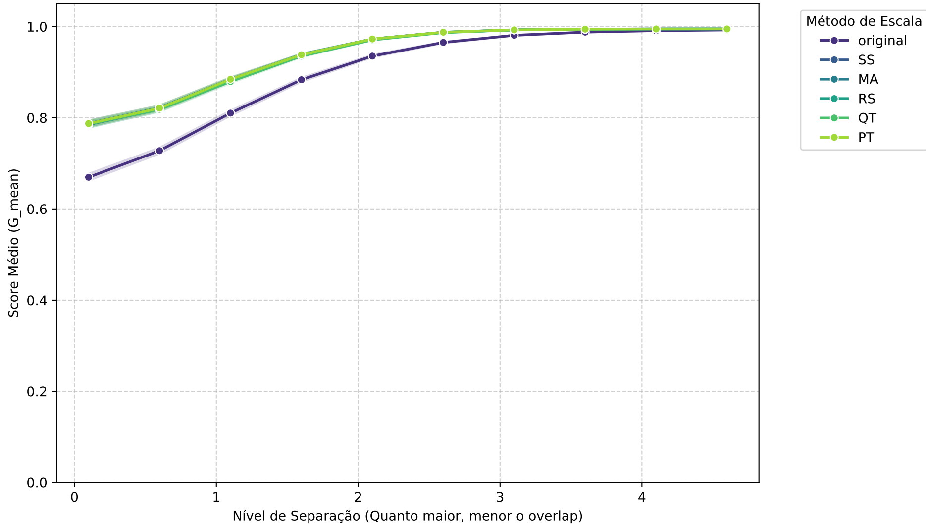
Média Geral: SVM_rbf - G_MEAN vs Separação
