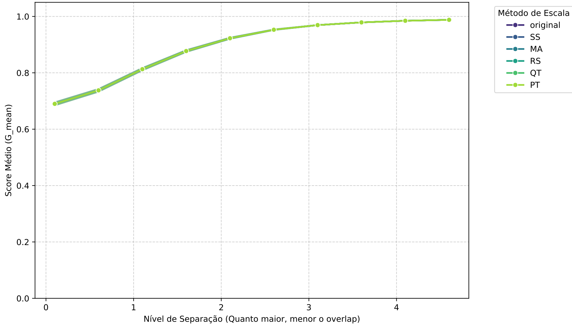
Média Geral: XGBoost - G_MEAN vs Separação
