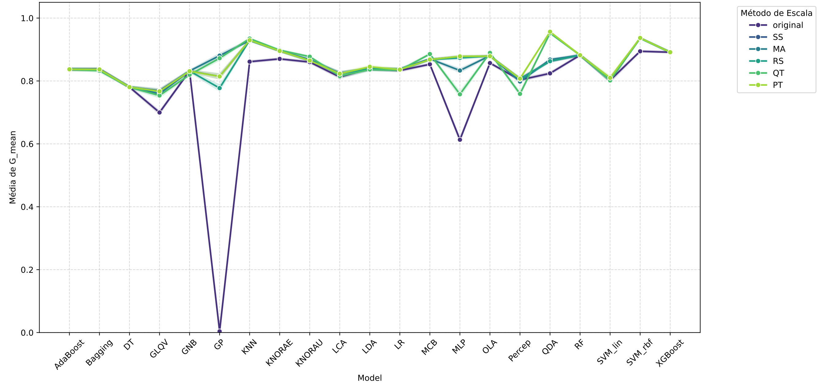
Média Global (Tendência por Modelo) - G_MEAN
