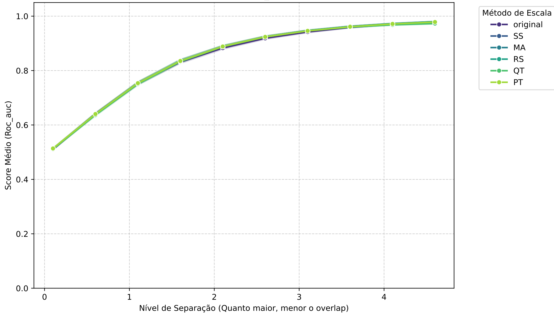
Média Geral: Bagging - ROC_AUC vs Separação
