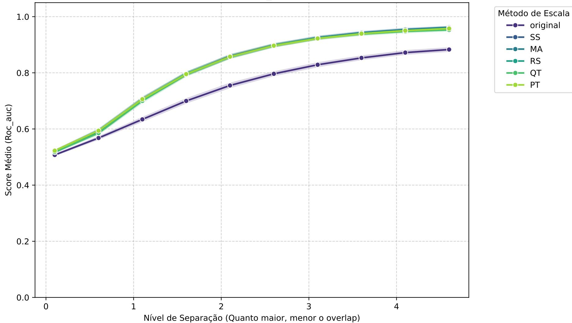
Média Geral: GLQV - ROC_AUC vs Separação
