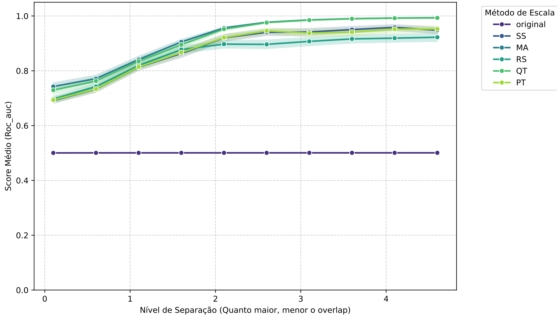
Média Geral: GP - ROC_AUC vs Separação
