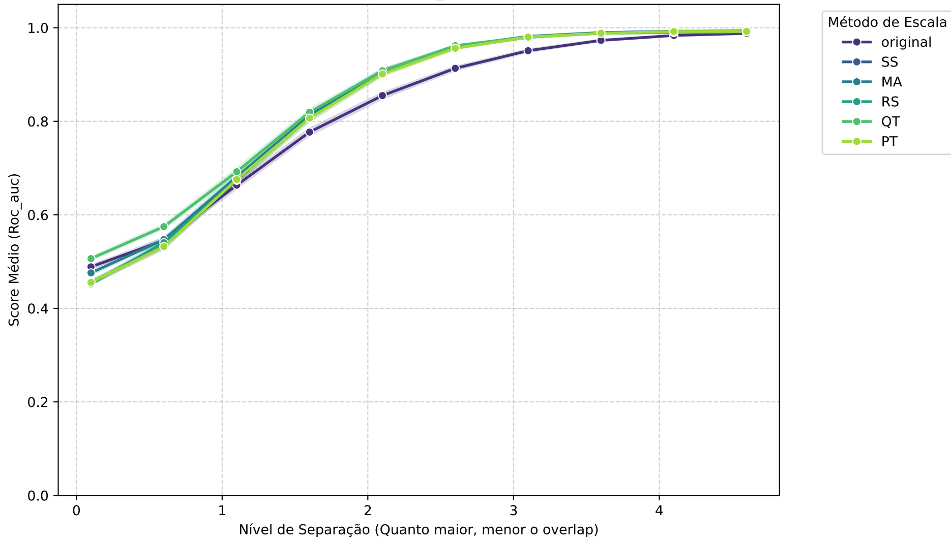
Média Geral: LCA - ROC_AUC vs Separação
