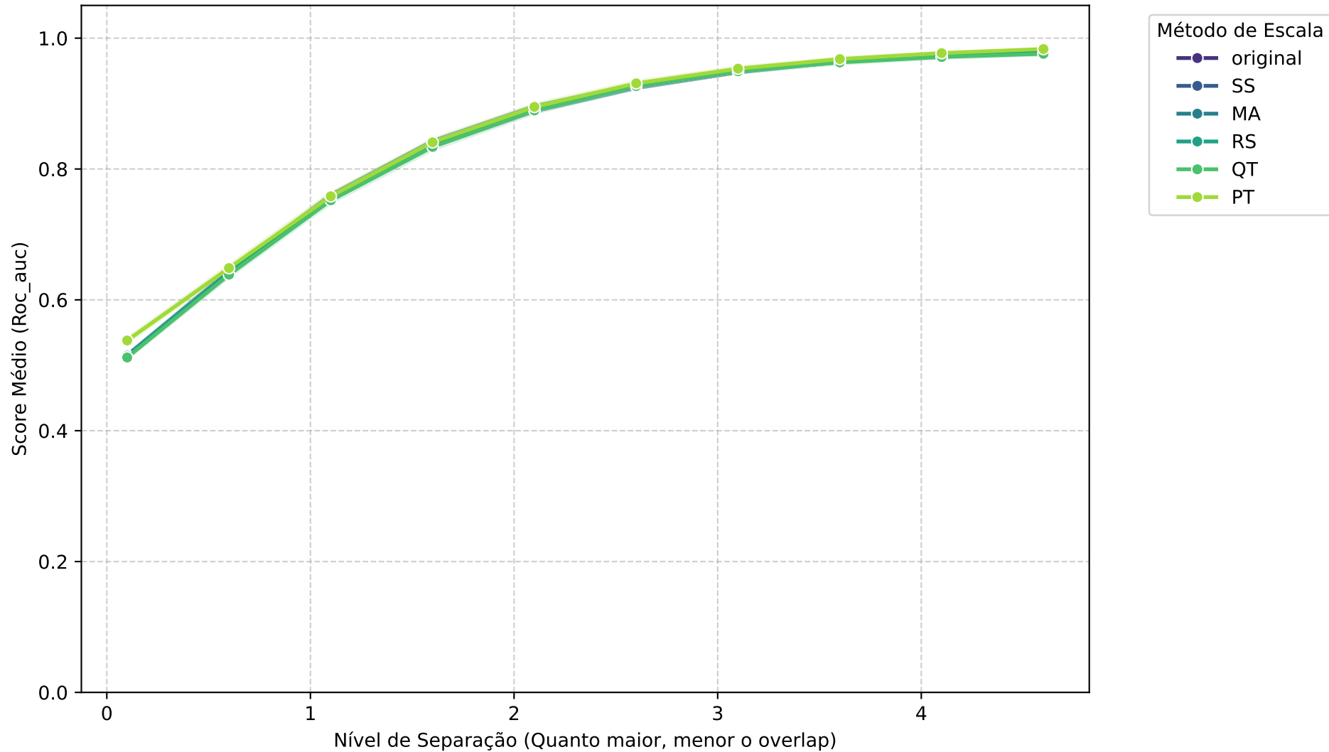
Média Geral: LDA - ROC_AUC vs Separação
