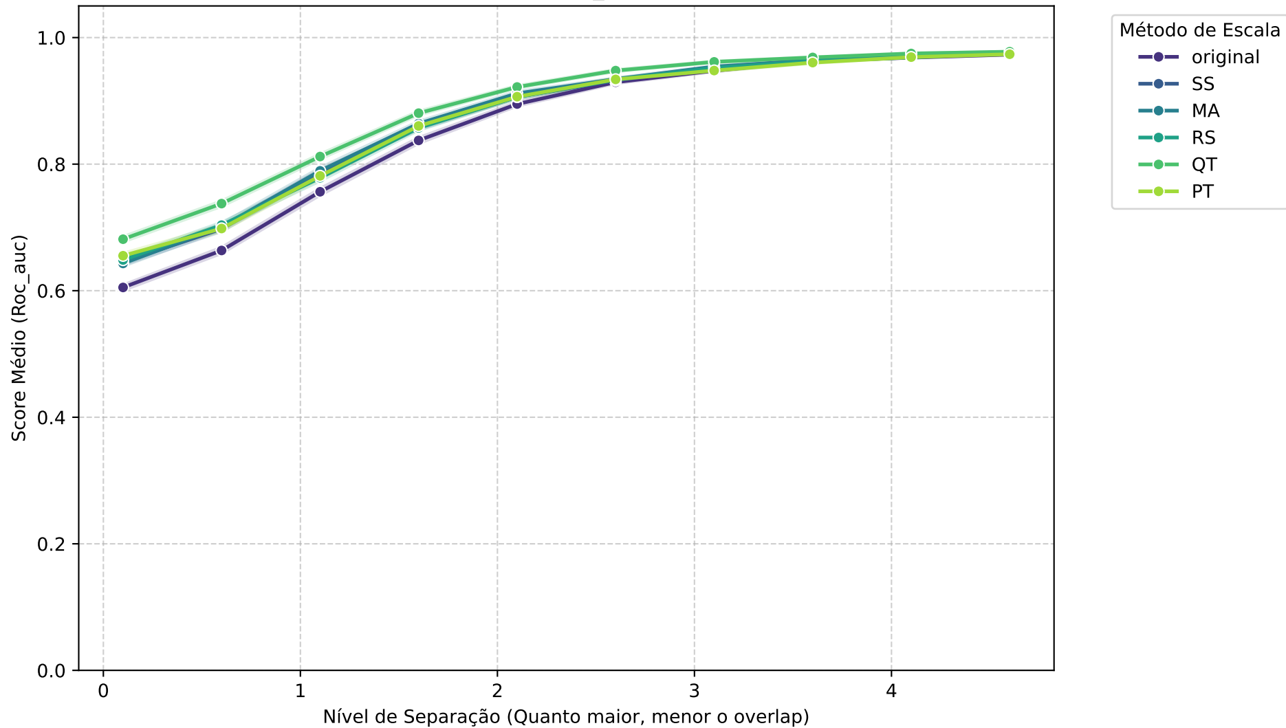
Média Geral: MCB - ROC_AUC vs Separação
