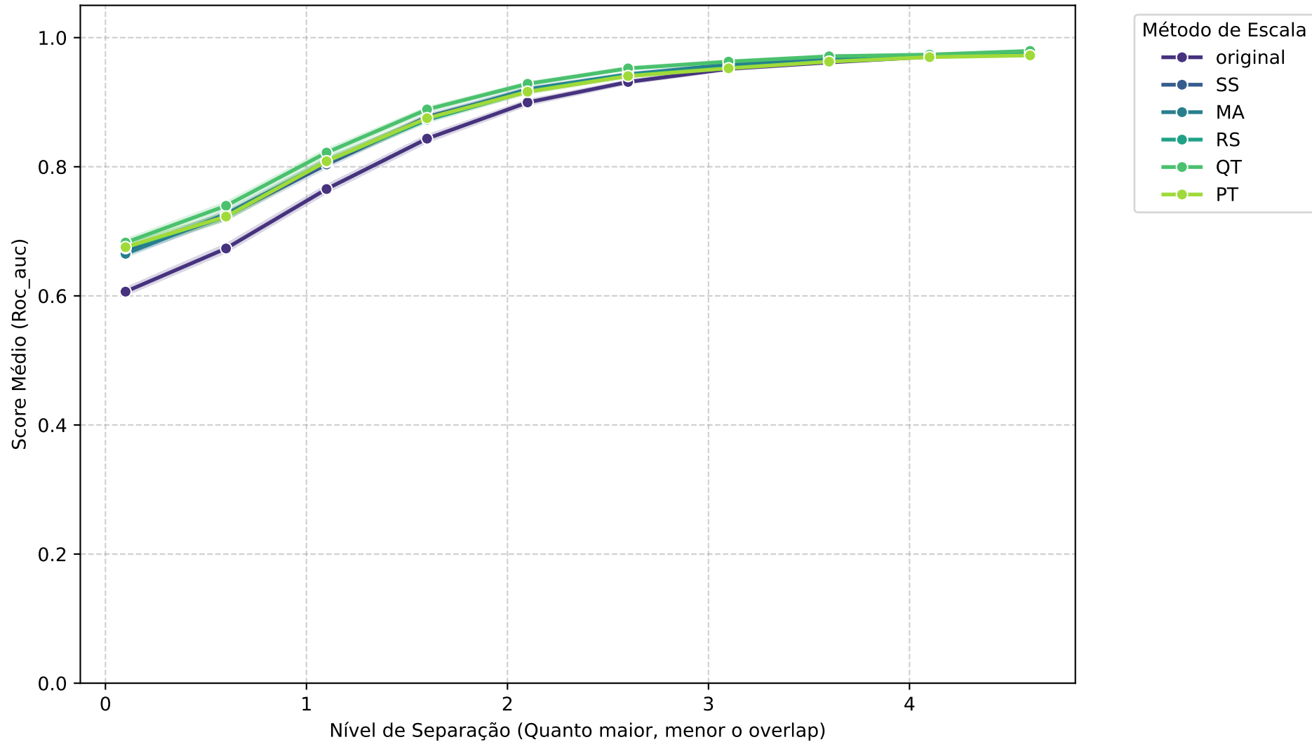
Média Geral: OLA - ROC_AUC vs Separação
