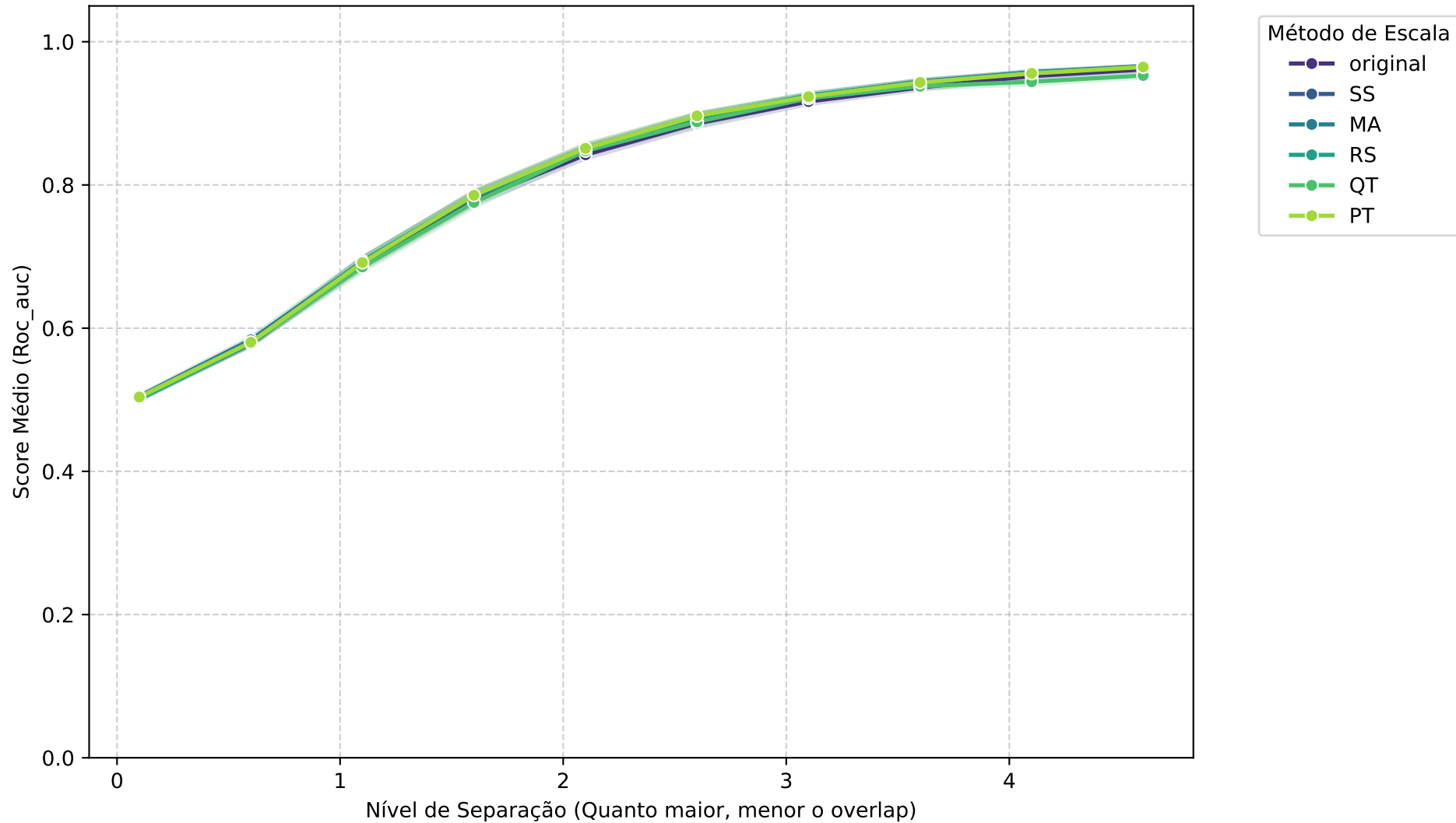
Média Geral: Percep - ROC_AUC vs Separação
