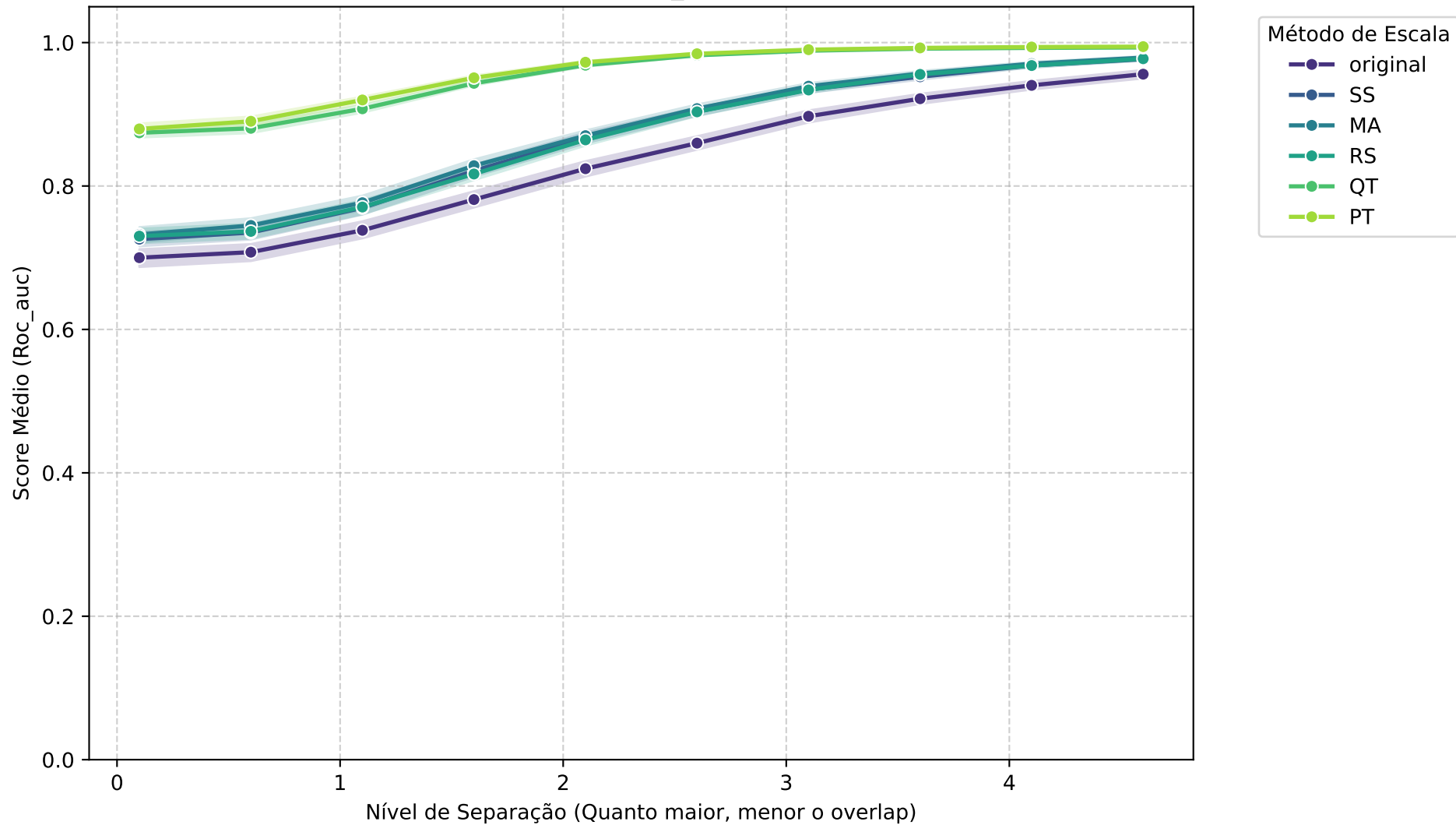
Média Geral: QDA - ROC_AUC vs Separação
