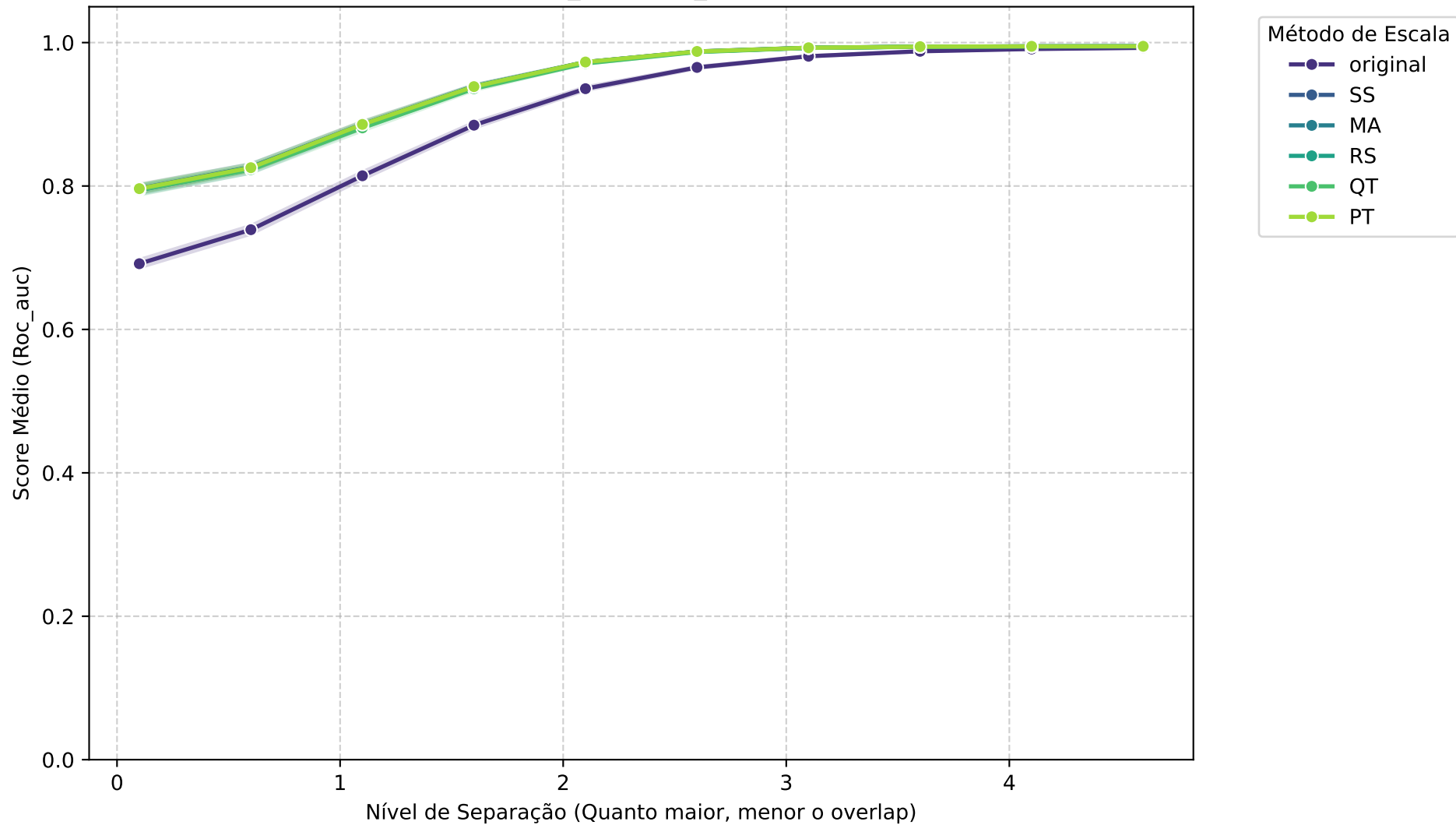
Média Geral: SVM_rbf - ROC_AUC vs Separação
