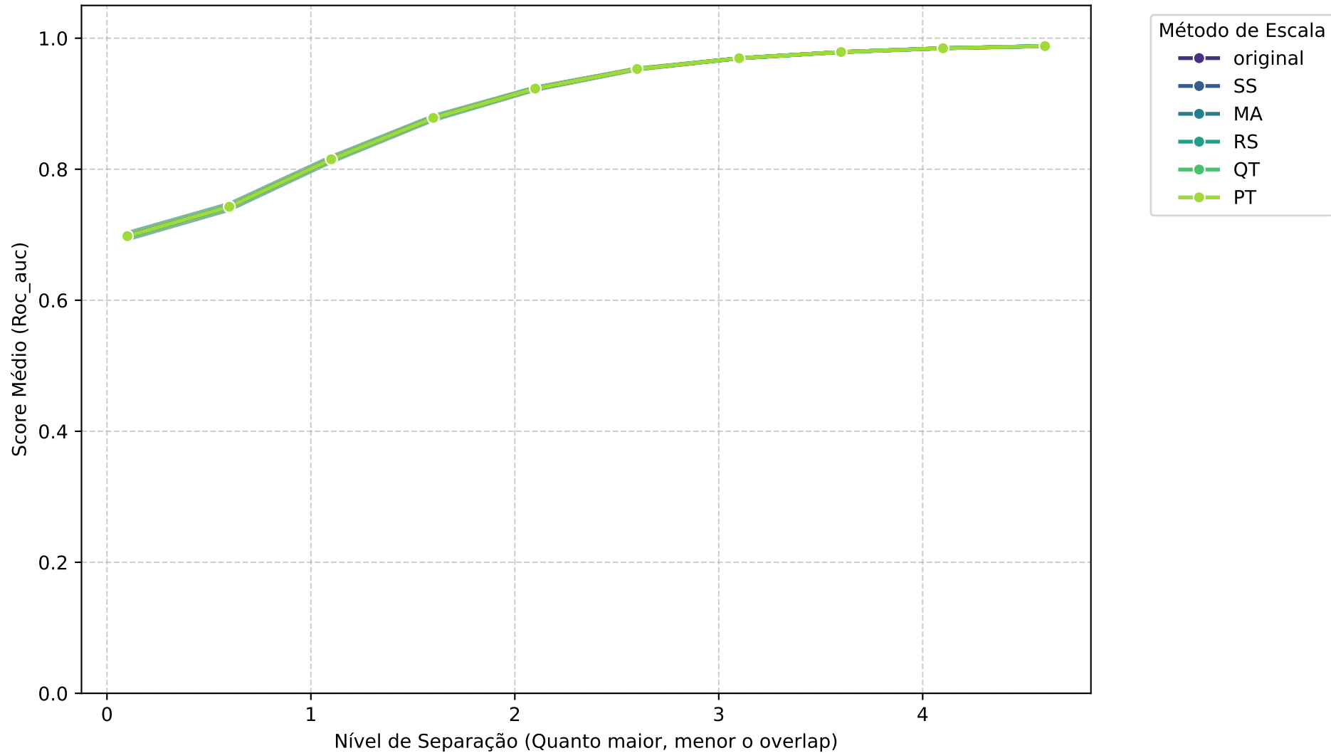
Média Geral: XGBoost - ROC_AUC vs Separação
