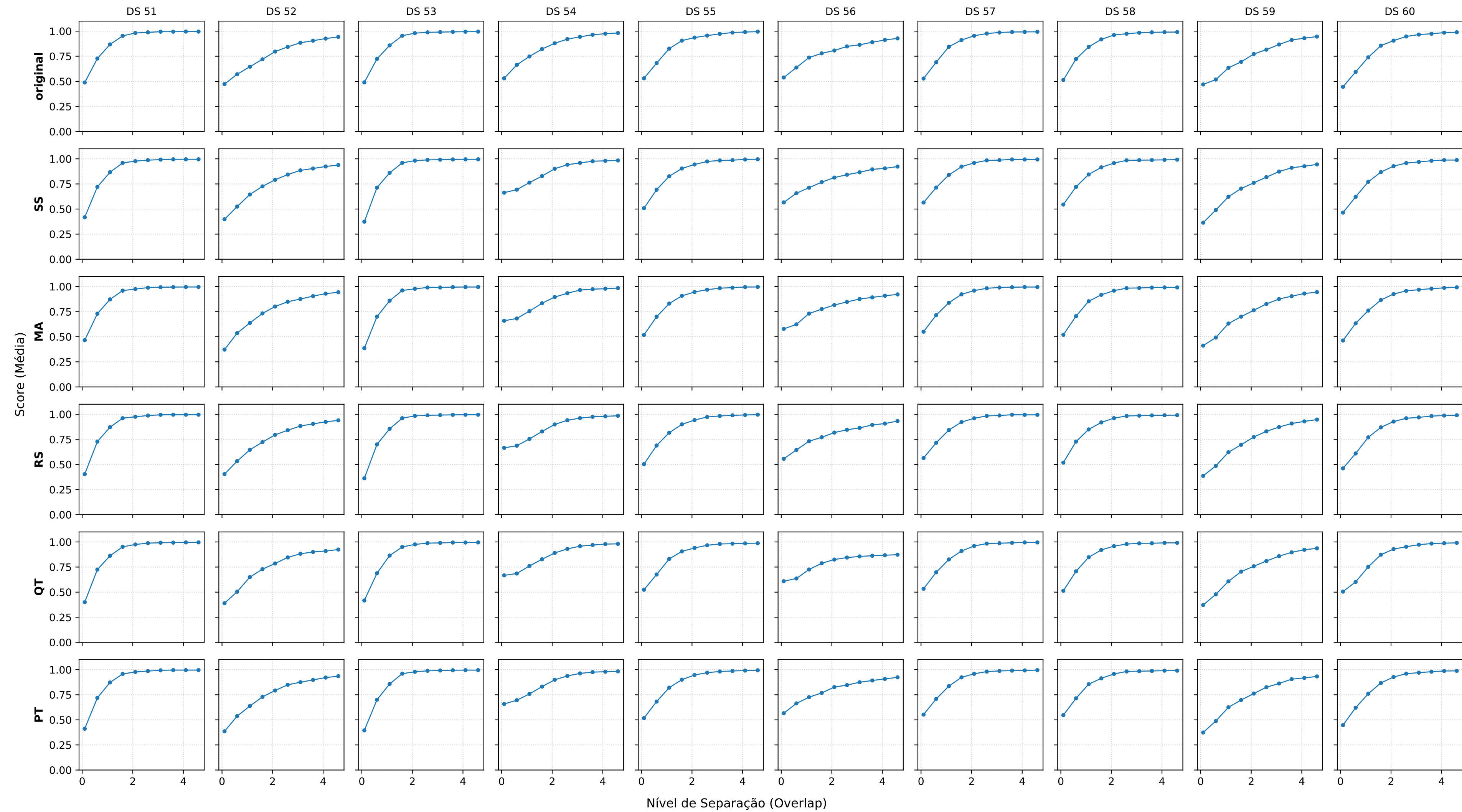
Modelo: Bagging | Métrica: F1_SCORE | Datasets: 51-60
