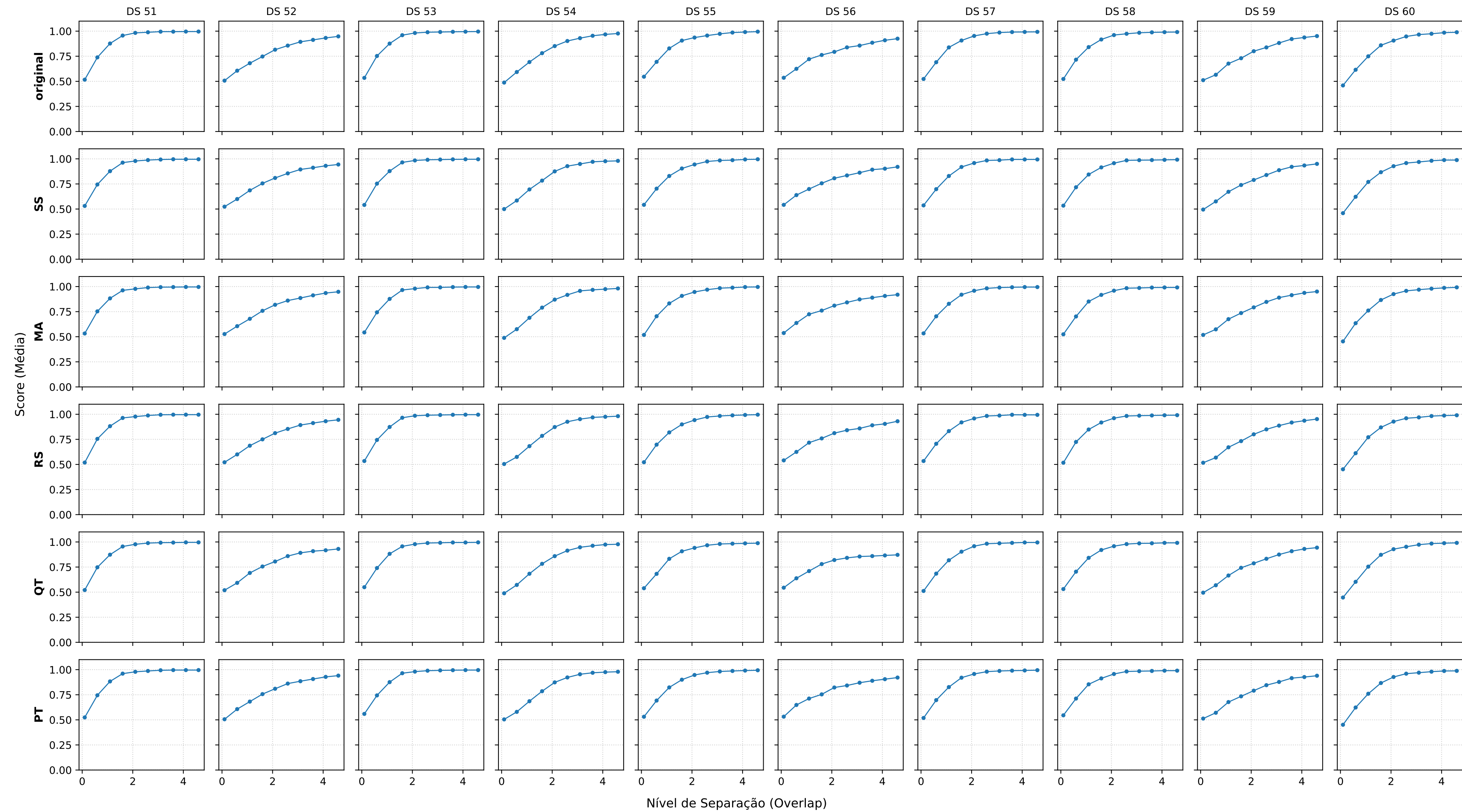
Modelo: Bagging | Métrica: ROC_AUC | Datasets: 51-60
