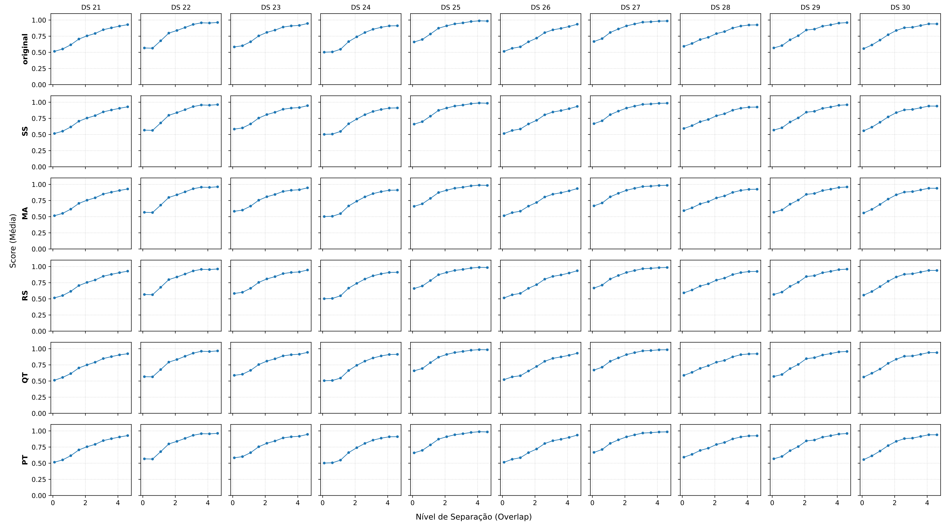
Modelo: DT | Métrica: F1_SCORE | Datasets: 21-30
