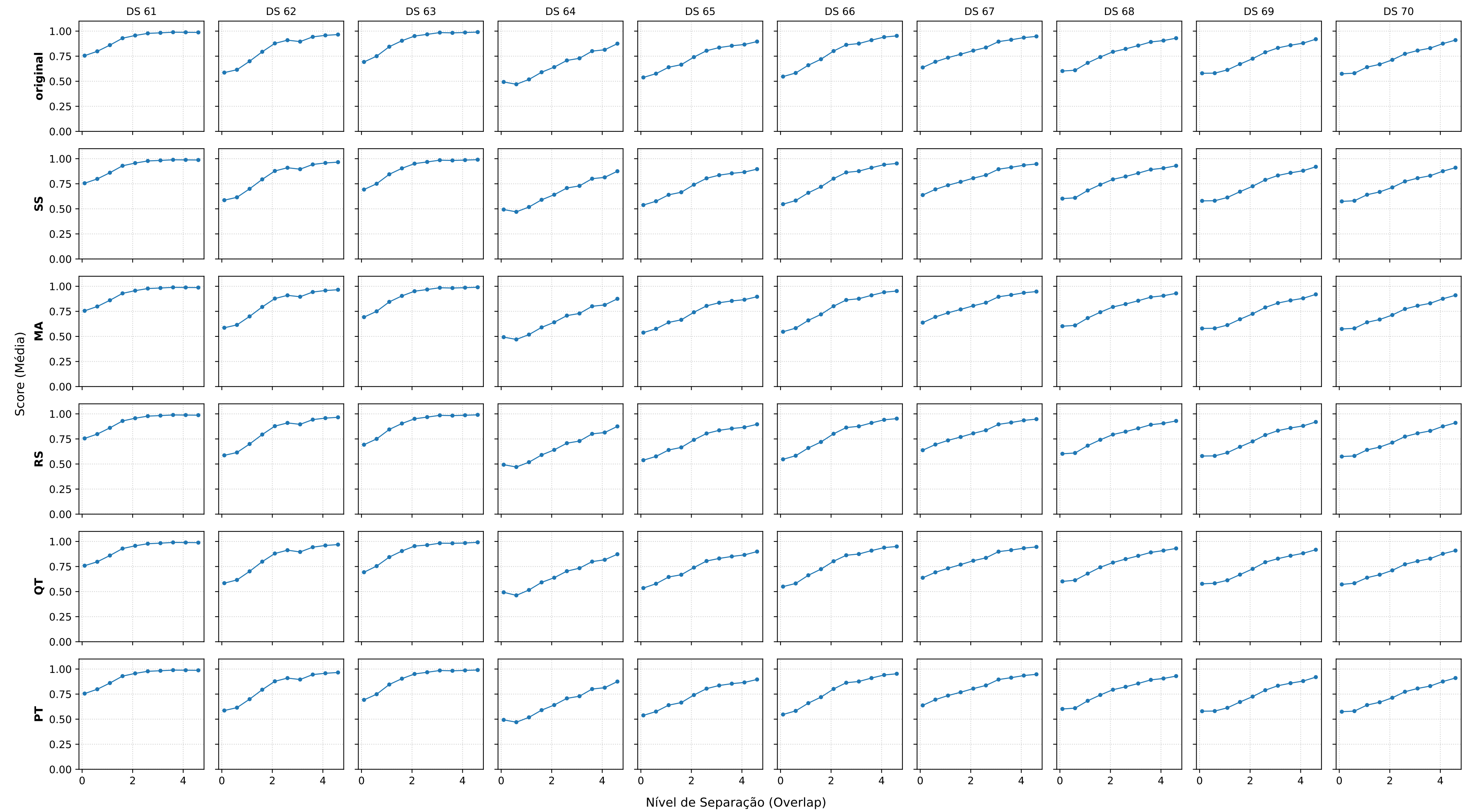
Modelo: DT | Métrica: F1_SCORE | Datasets: 61-70
