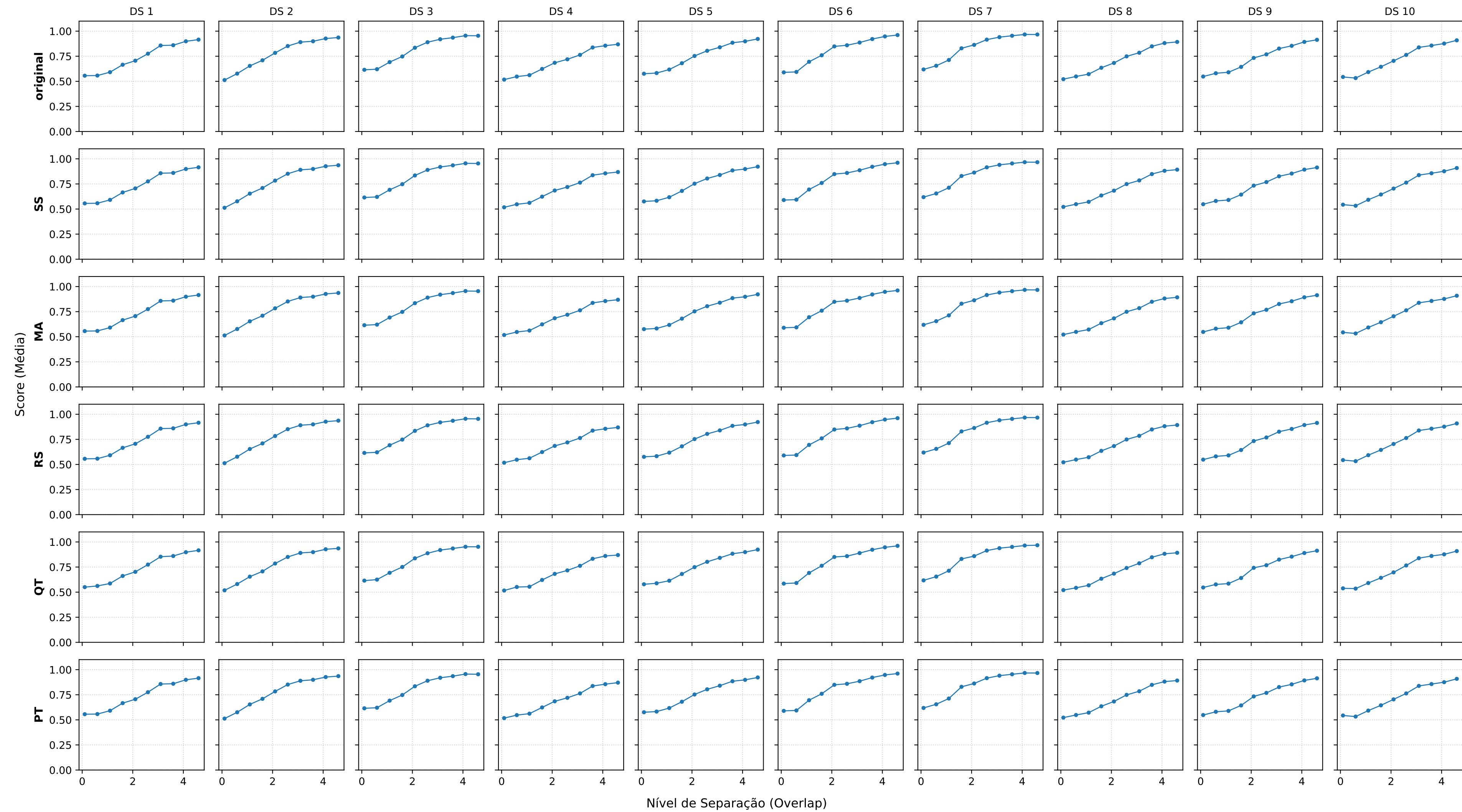
Modelo: DT | Métrica: G_MEAN | Datasets: 1-10
