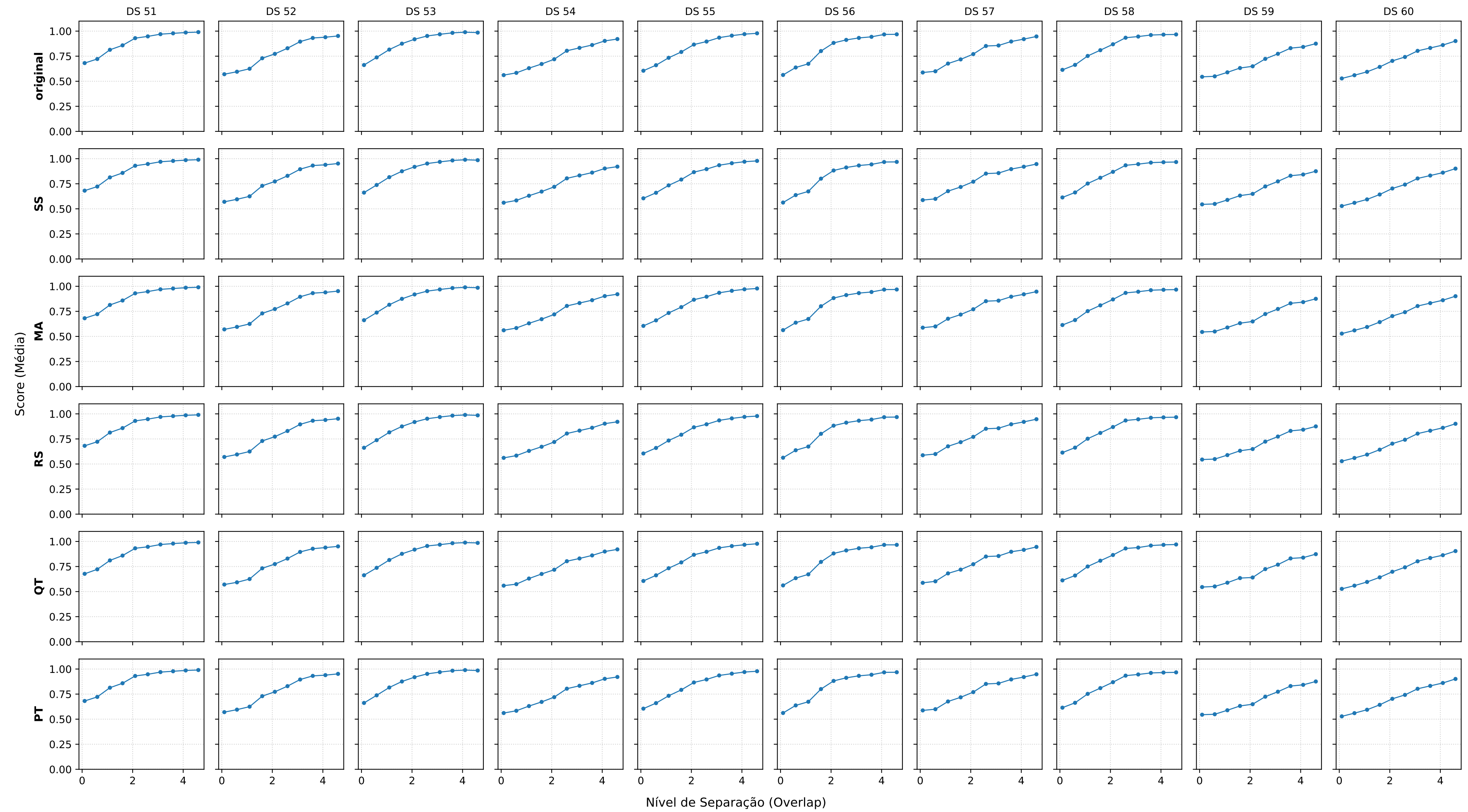
Modelo: DT | Métrica: ROC_AUC | Datasets: 51-60
