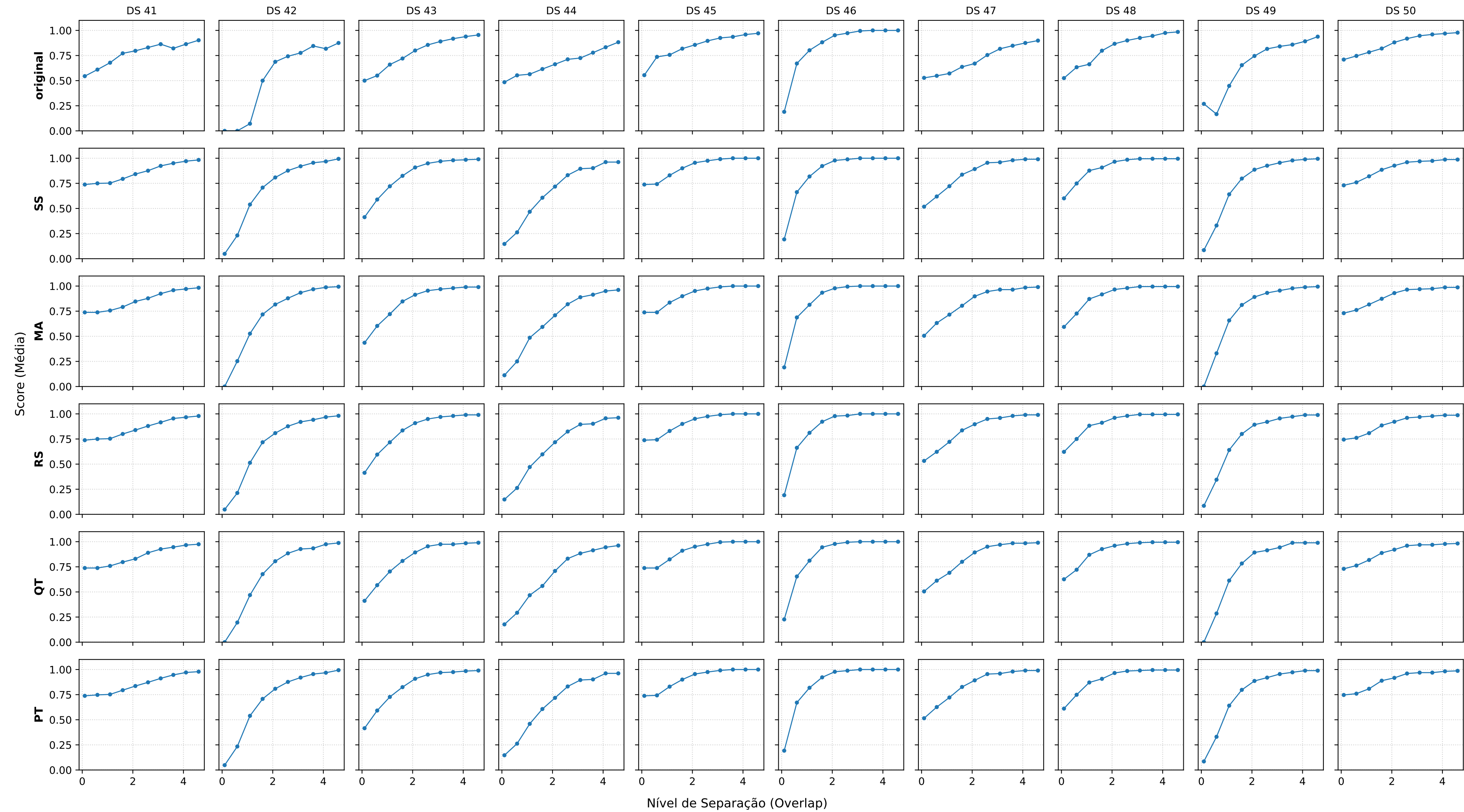
Modelo: GLQV | Métrica: F1_SCORE | Datasets: 41-50
