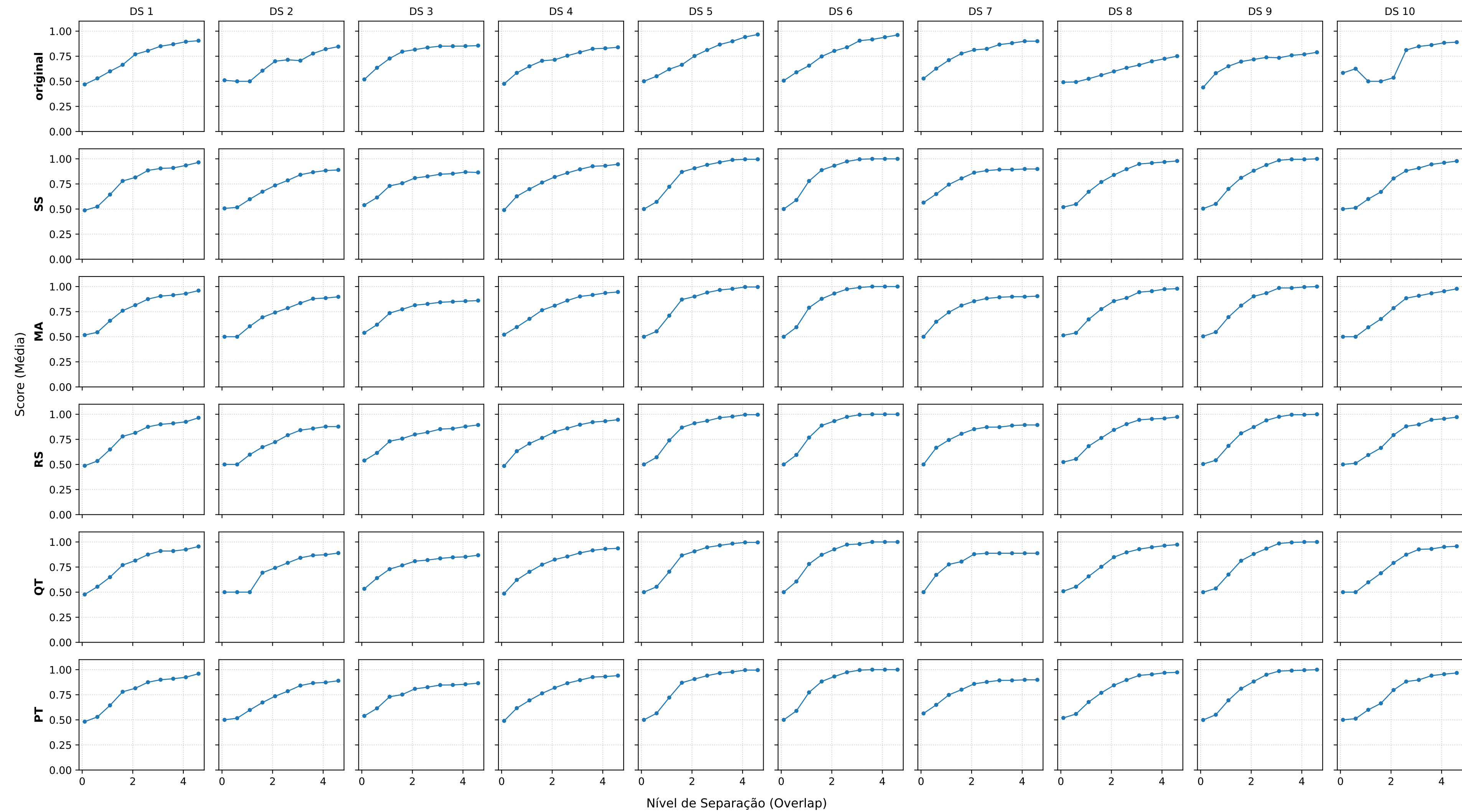
Modelo: GLQV | Métrica: ROC_AUC | Datasets: 1-10
