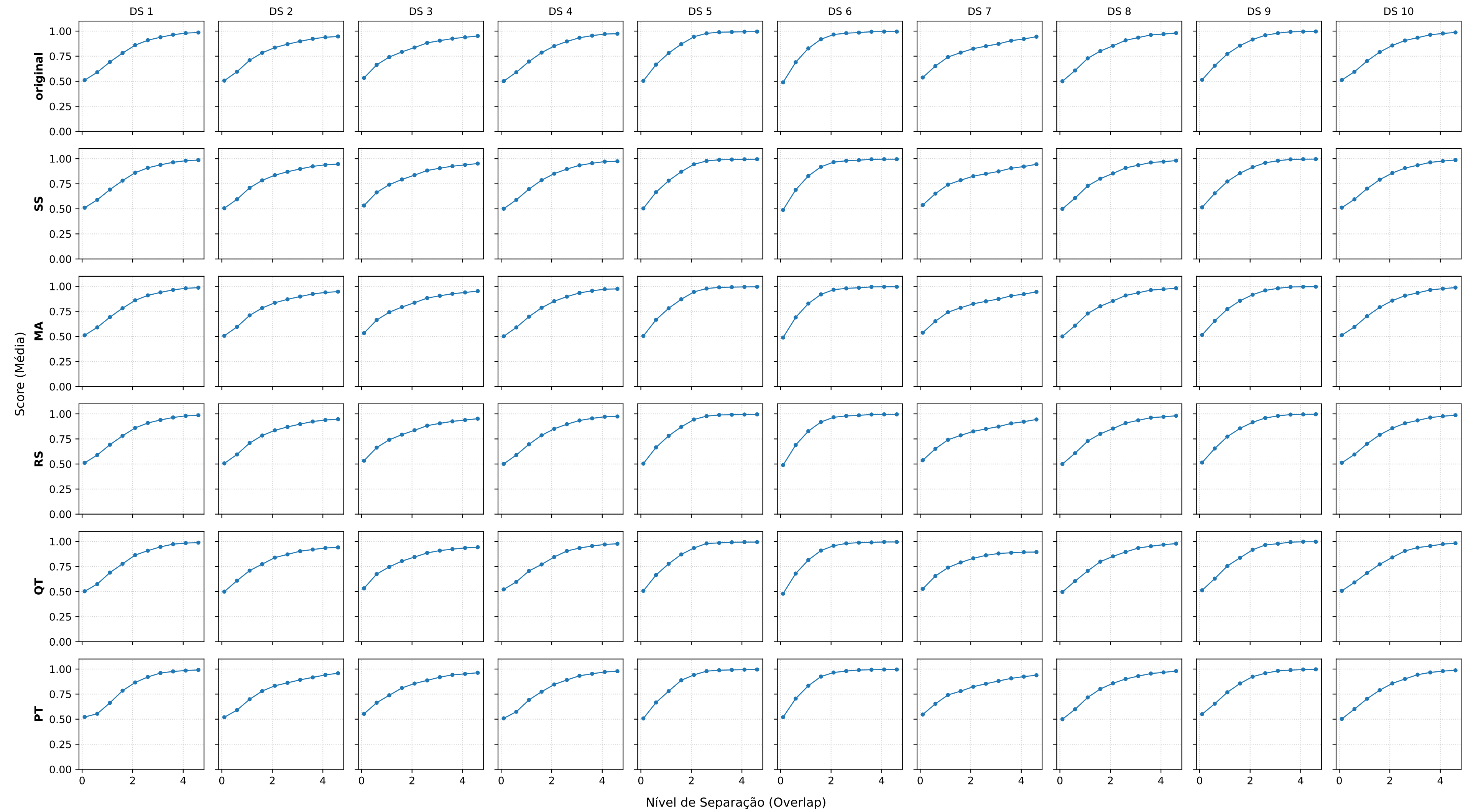
Modelo: LDA | Métrica: ROC_AUC | Datasets: 1-10
