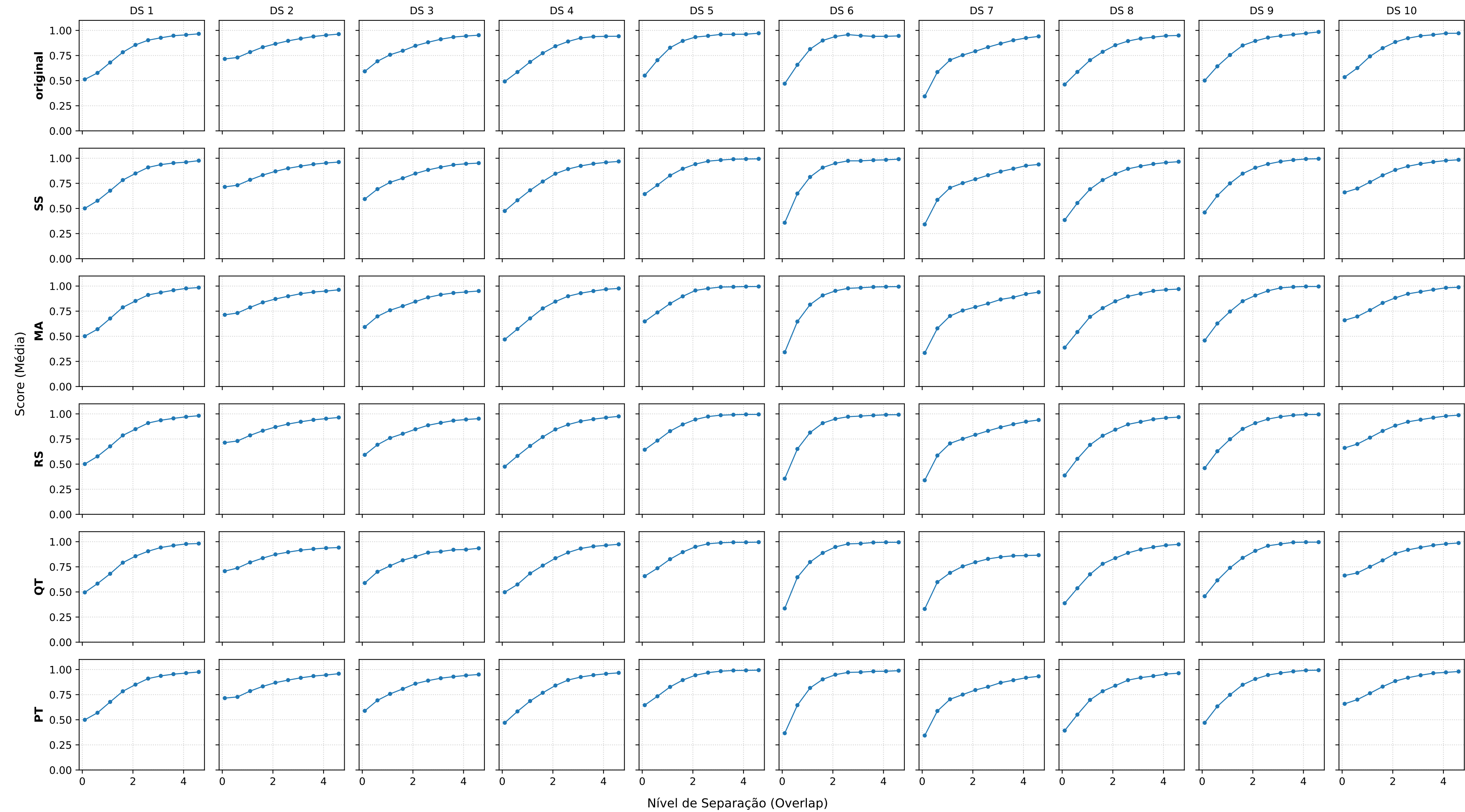
Modelo: LR | Métrica: F1_SCORE | Datasets: 1-10
