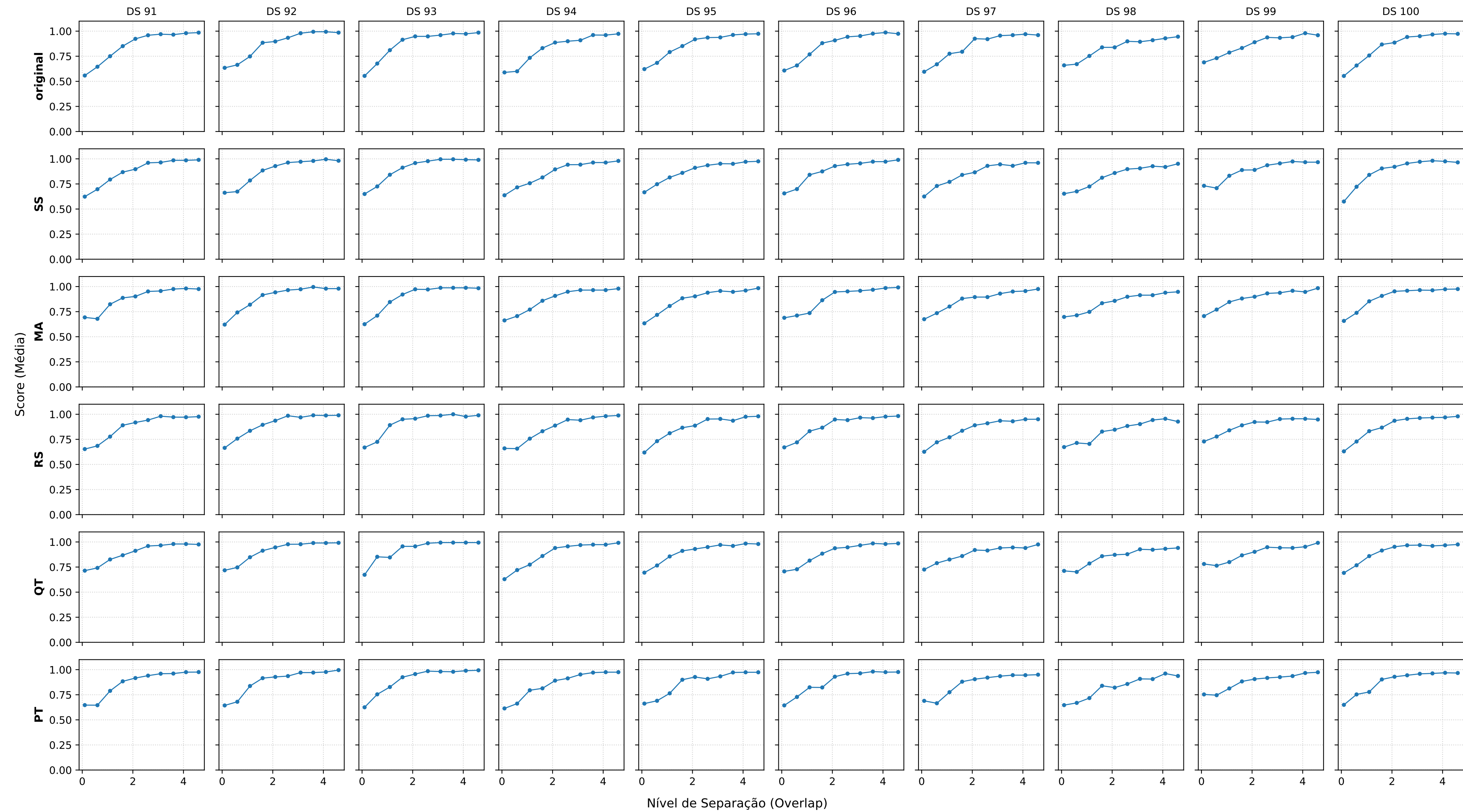
Modelo: MCB | Métrica: ROC_AUC | Datasets: 91-100
