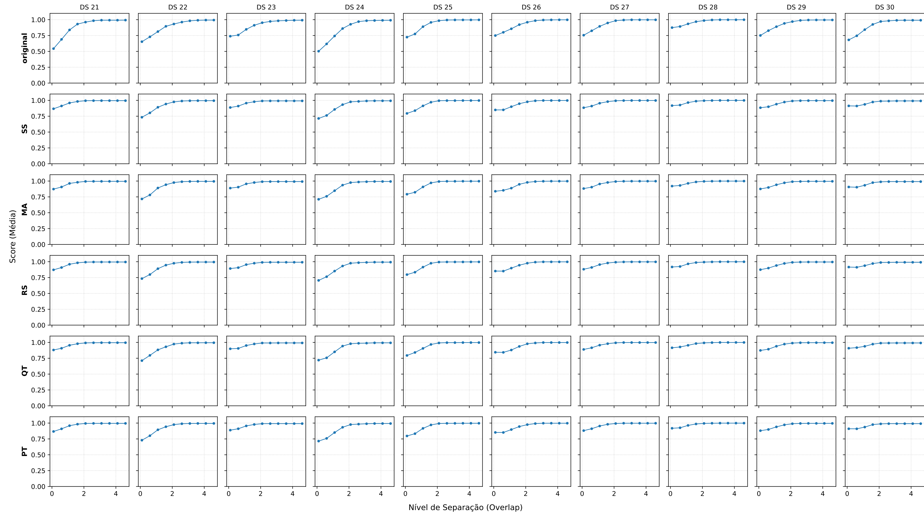
Modelo: SVM_rbf | Métrica: F1_SCORE | Datasets: 21-30
