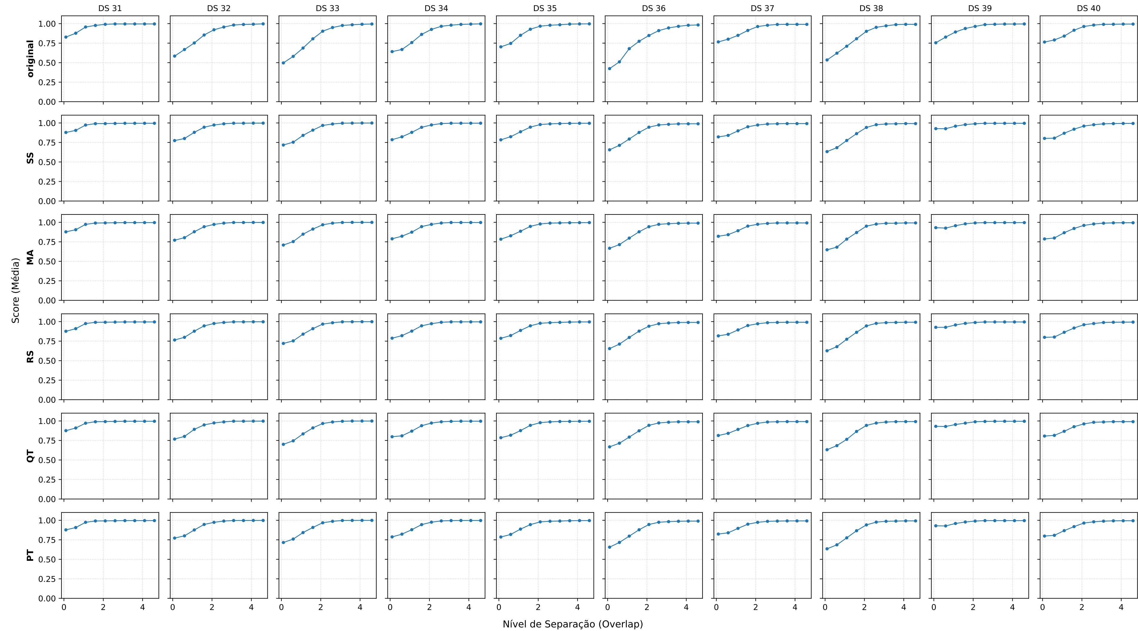
Modelo: SVM_rbf | Métrica: G_MEAN | Datasets: 31-40
