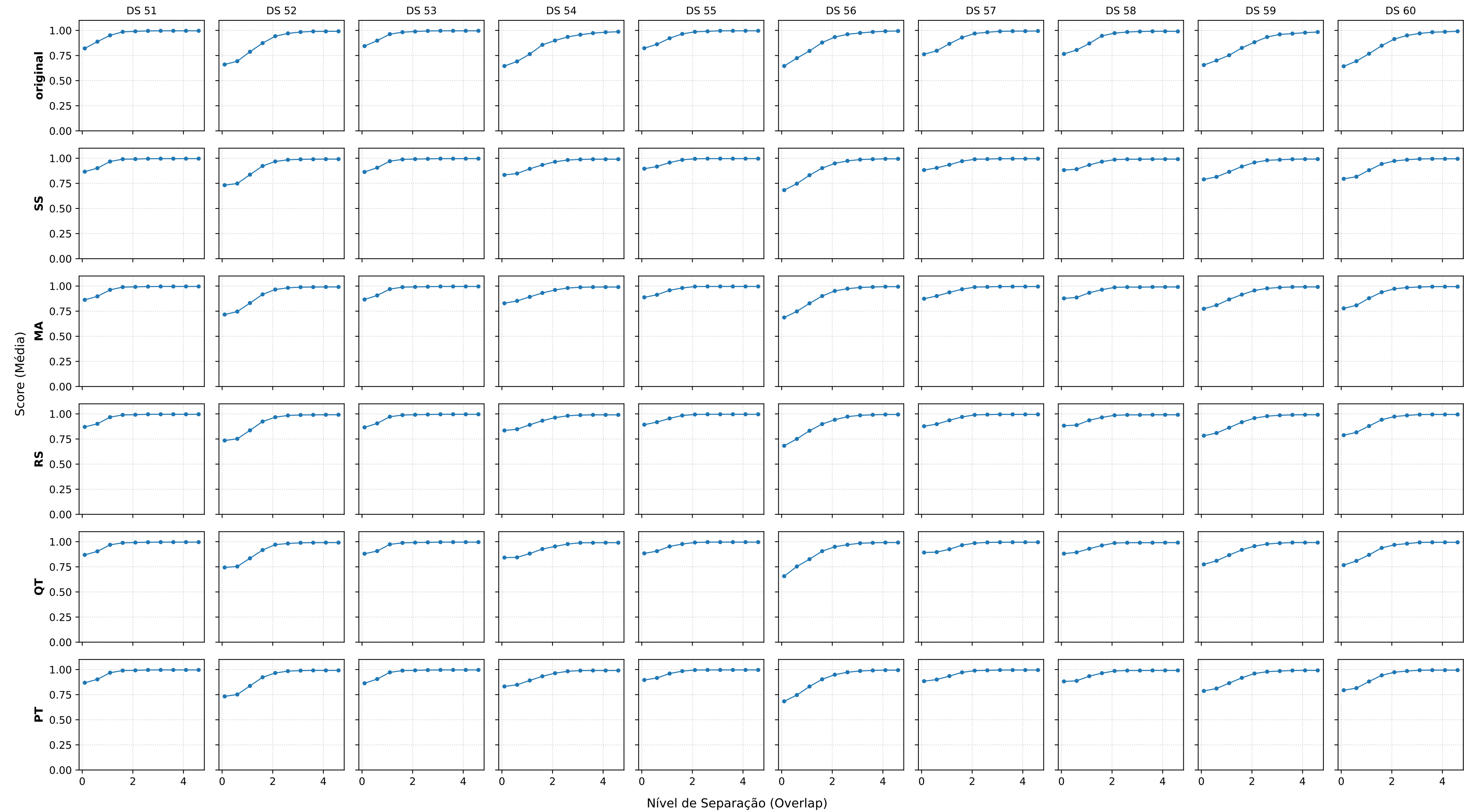
Modelo: SVM_rbf | Métrica: ROC_AUC | Datasets: 51-60
