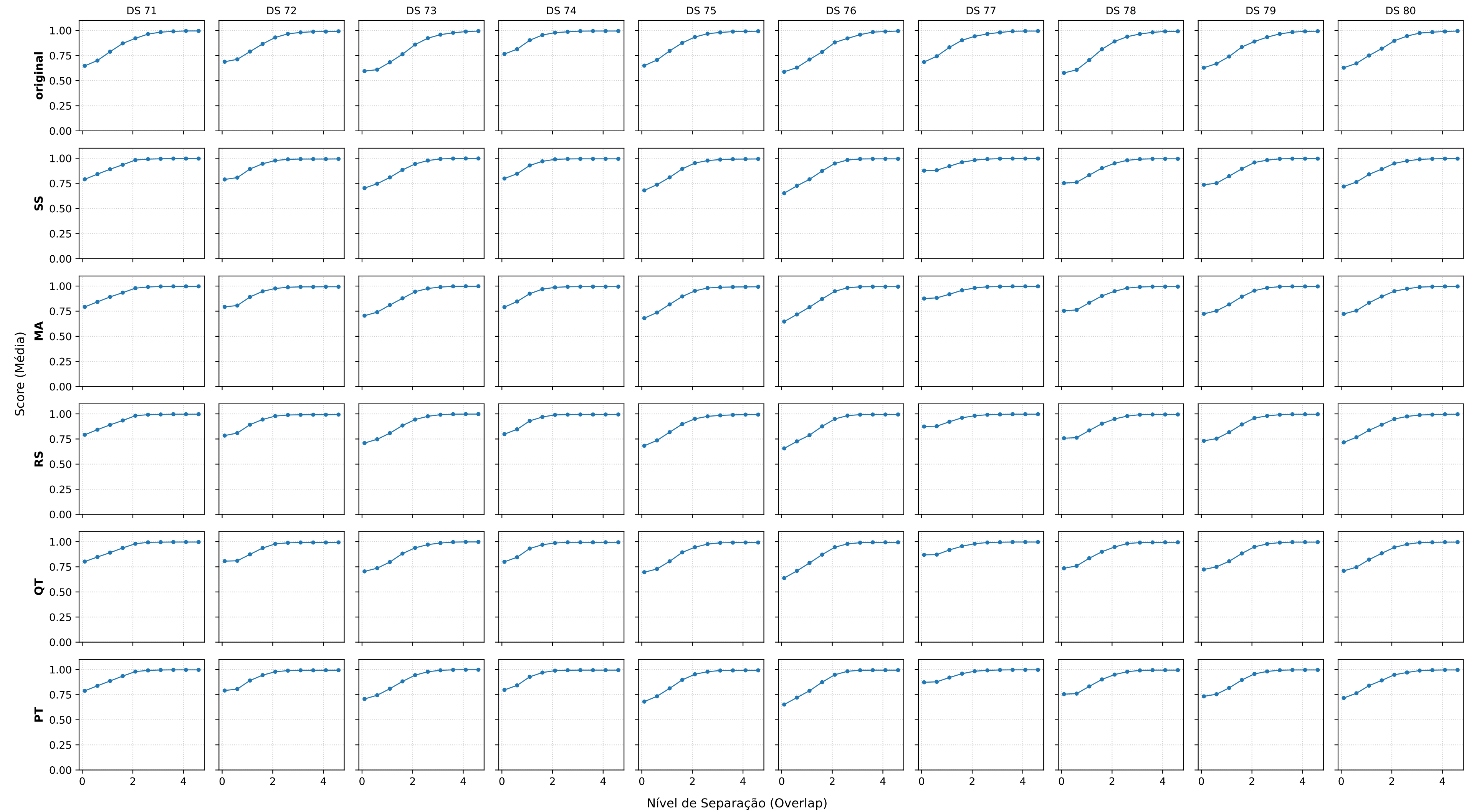
Modelo: SVM_rbf | Métrica: ROC_AUC | Datasets: 71-80
