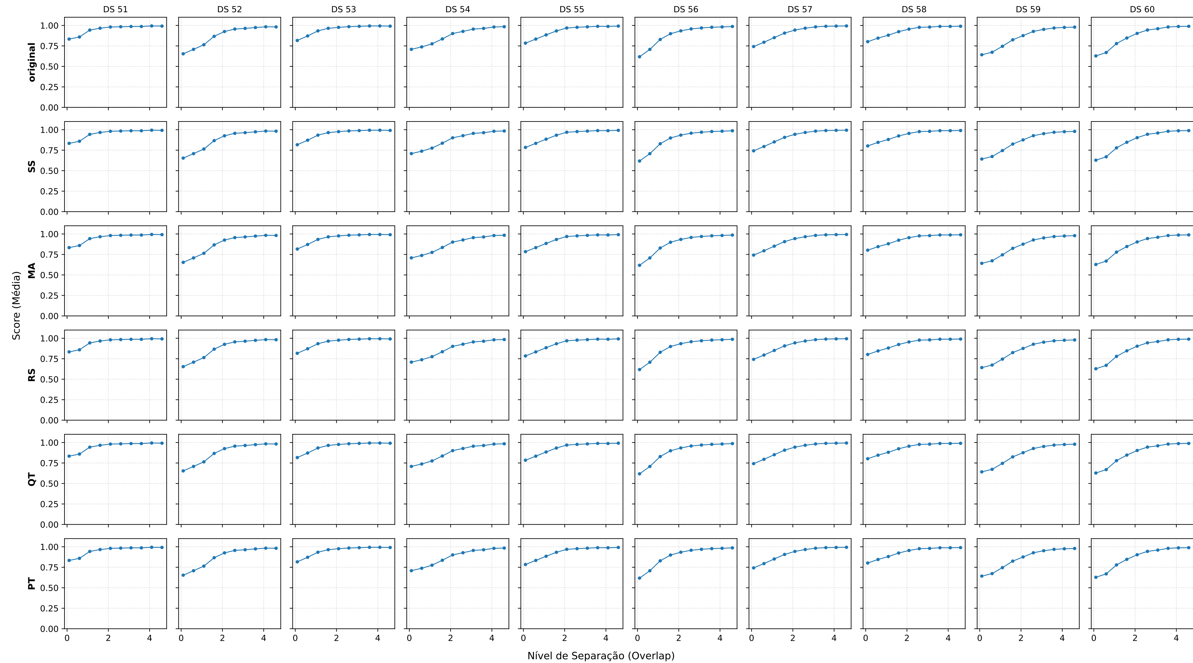
Modelo: XGBoost | Métrica: G_MEAN | Datasets: 51-60
