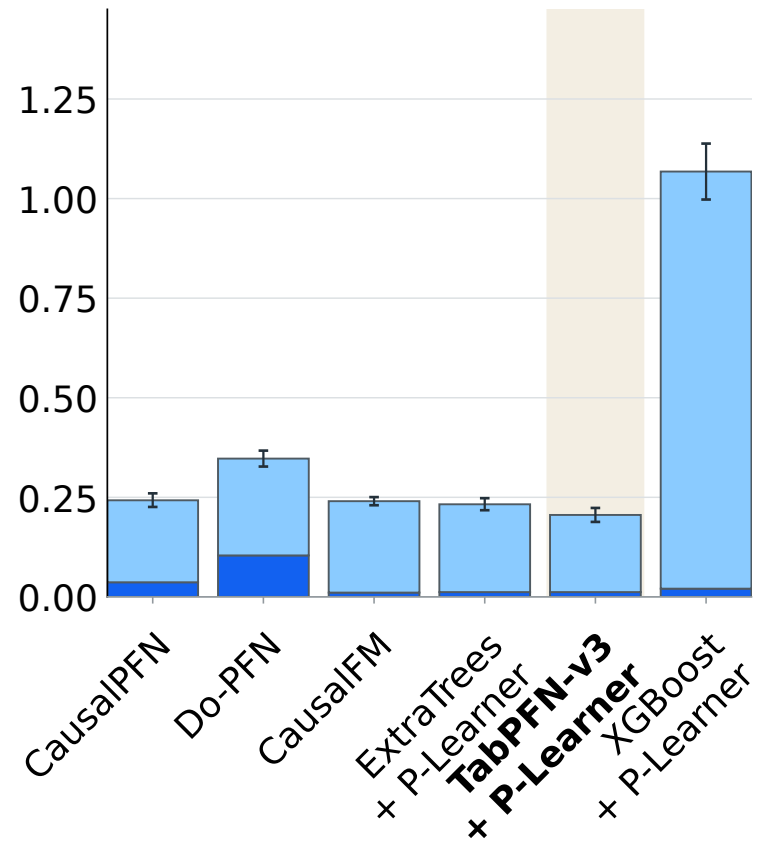
(d) Proximal
