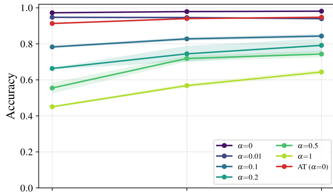
Purif. (lk., r=0.3 )
