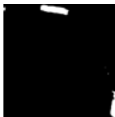
MCANet
