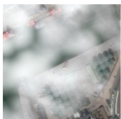
Degrade RGB
