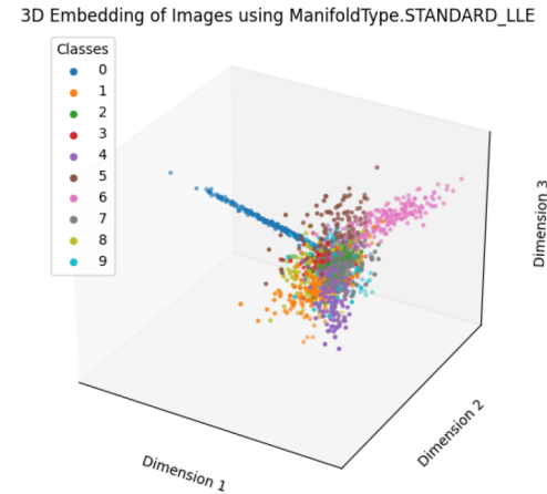
Standard LLE embedding (3D)
