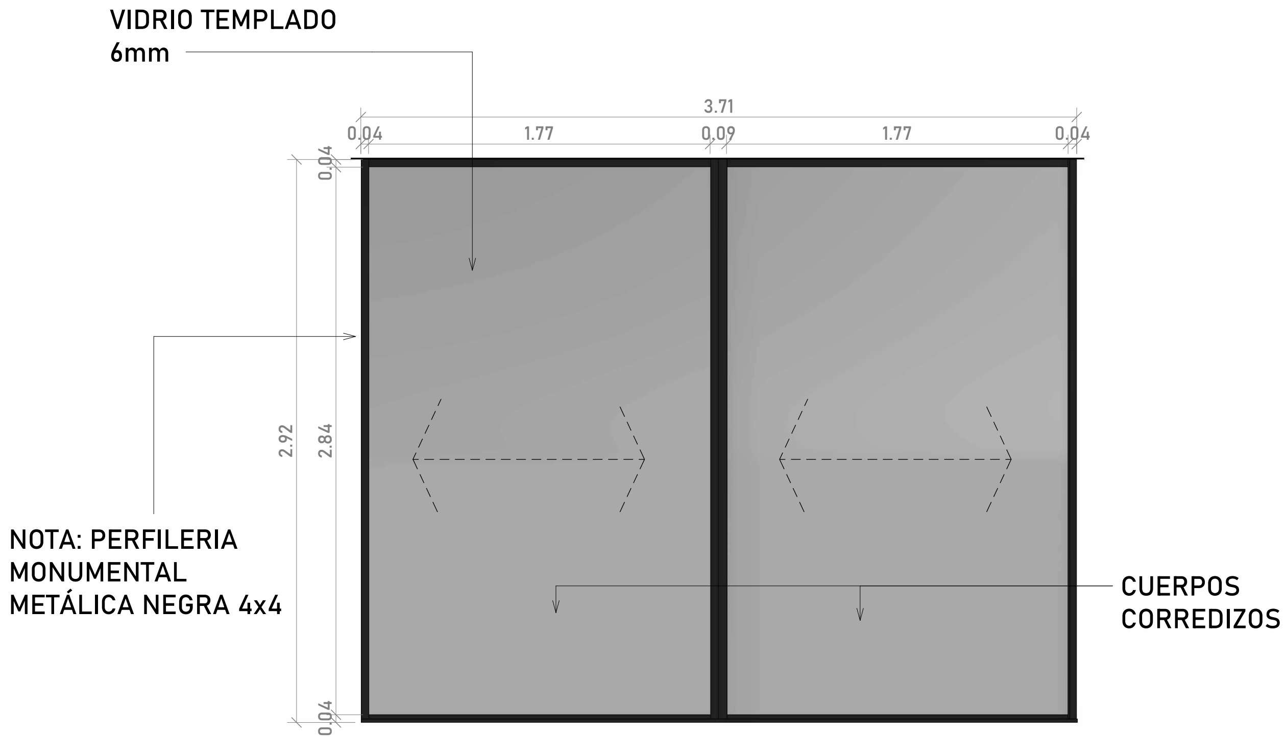
1 ALZADO VENTANA CORREDIZA SALA TV 1: 20
