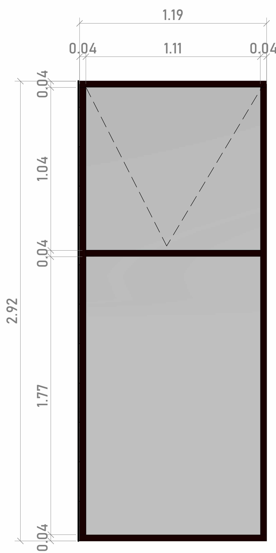
2 VENTANA DUCHA HABITACIÓN 3 1: 25
