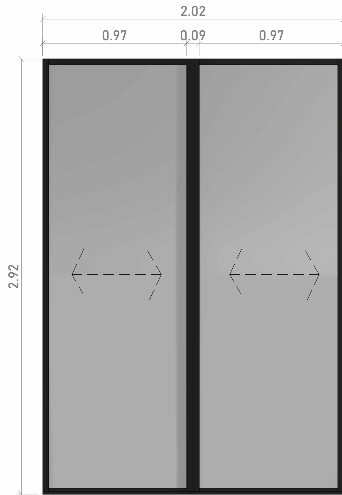
3 VIDRIERA CORREDIZA 2 HABITACIÓN PPAL 1: 25
