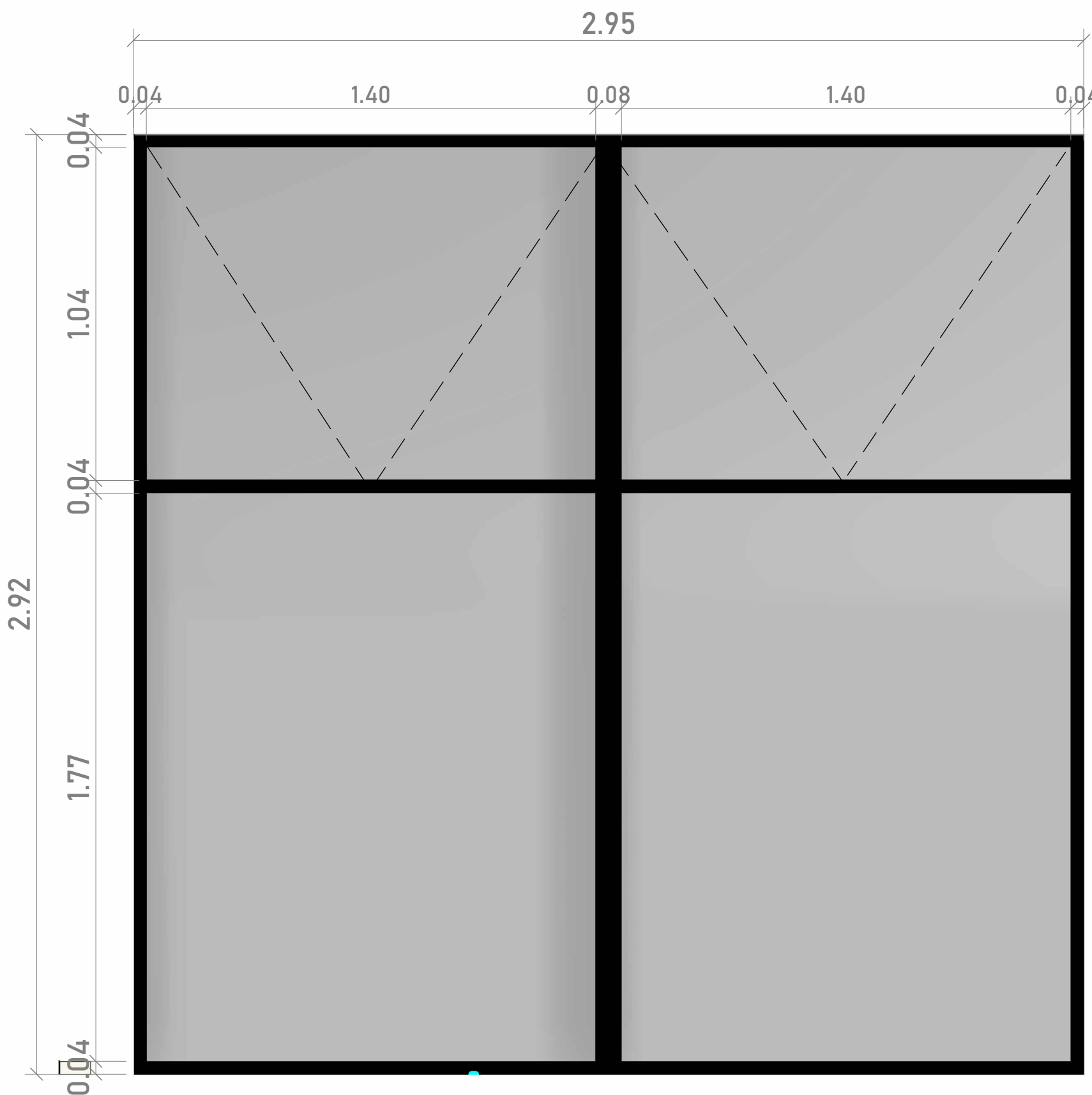
2 VENTANA DUCHA HABITACIÓN PPAL 1: 25
