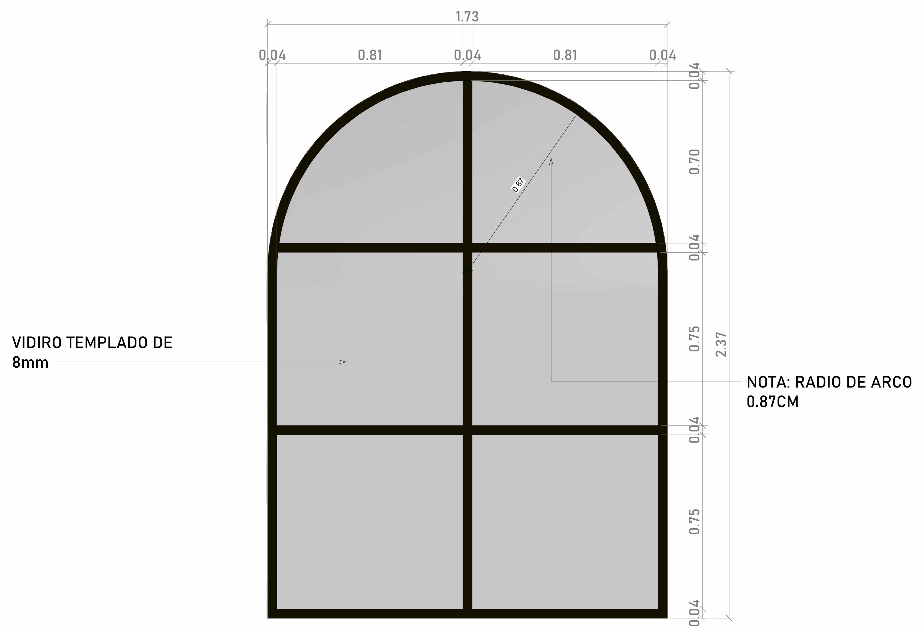
1 ALZADO ARCO PERFILERIA METÁLICA 1: 10
