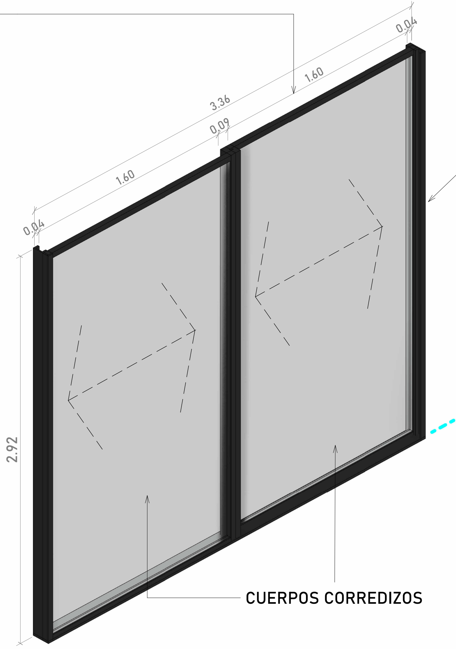
1 VENTANA CORREDIZA HABITACIÓN 2 1: 15
