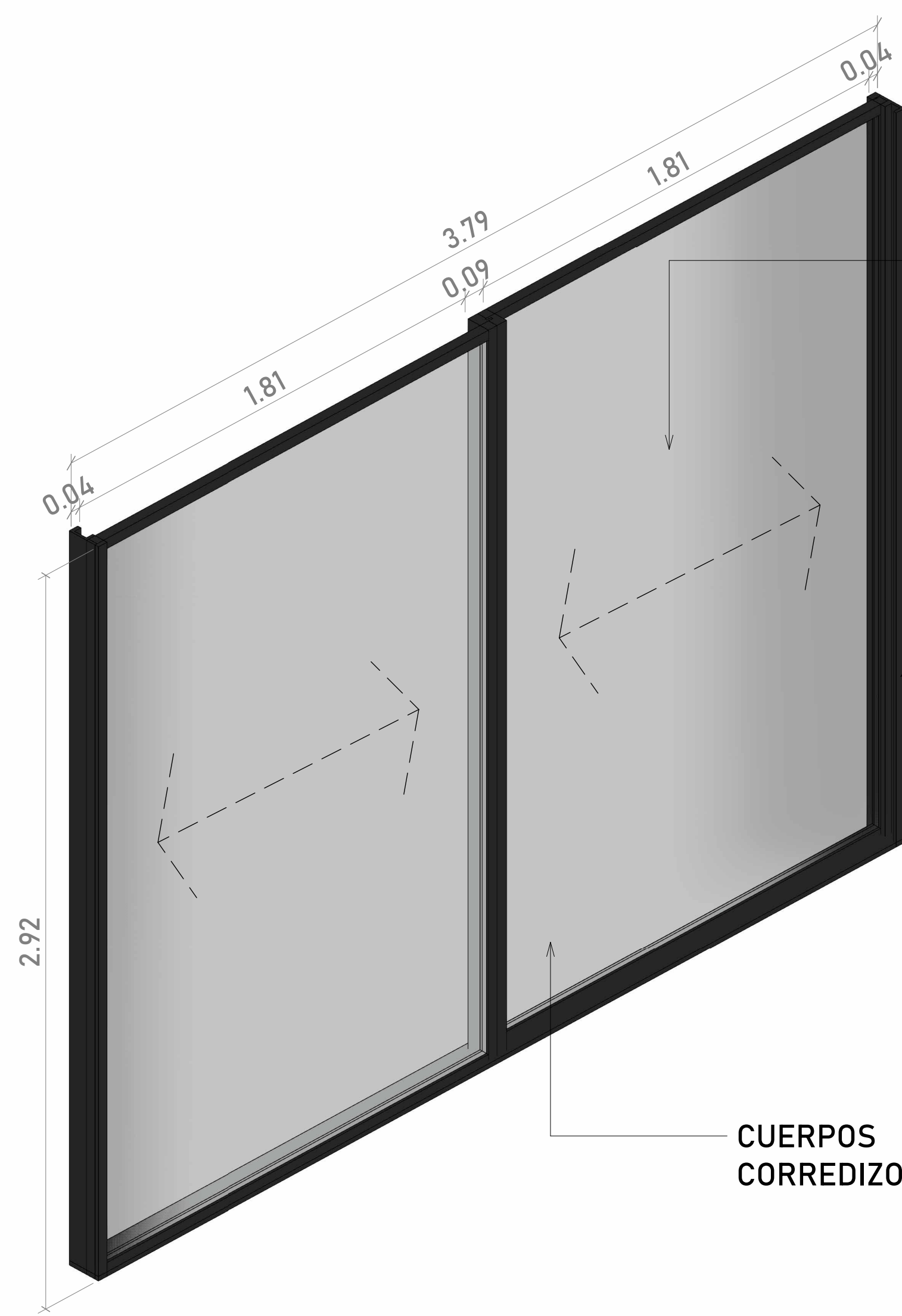
1 VENTANA CORREDIZA HABITACIÓN 3 1: 25
