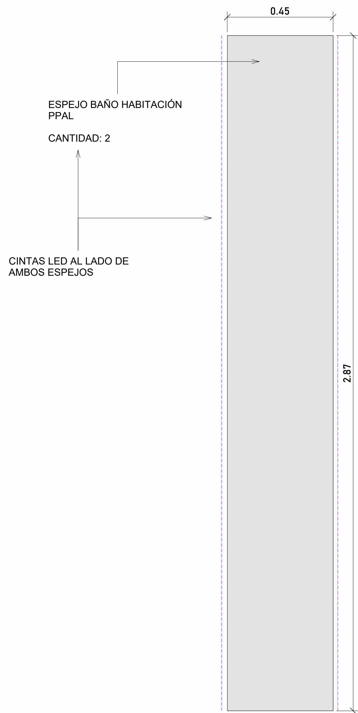
3 ESPEJO BAÑO HABITACIÓN PPAL ESC 1:10
