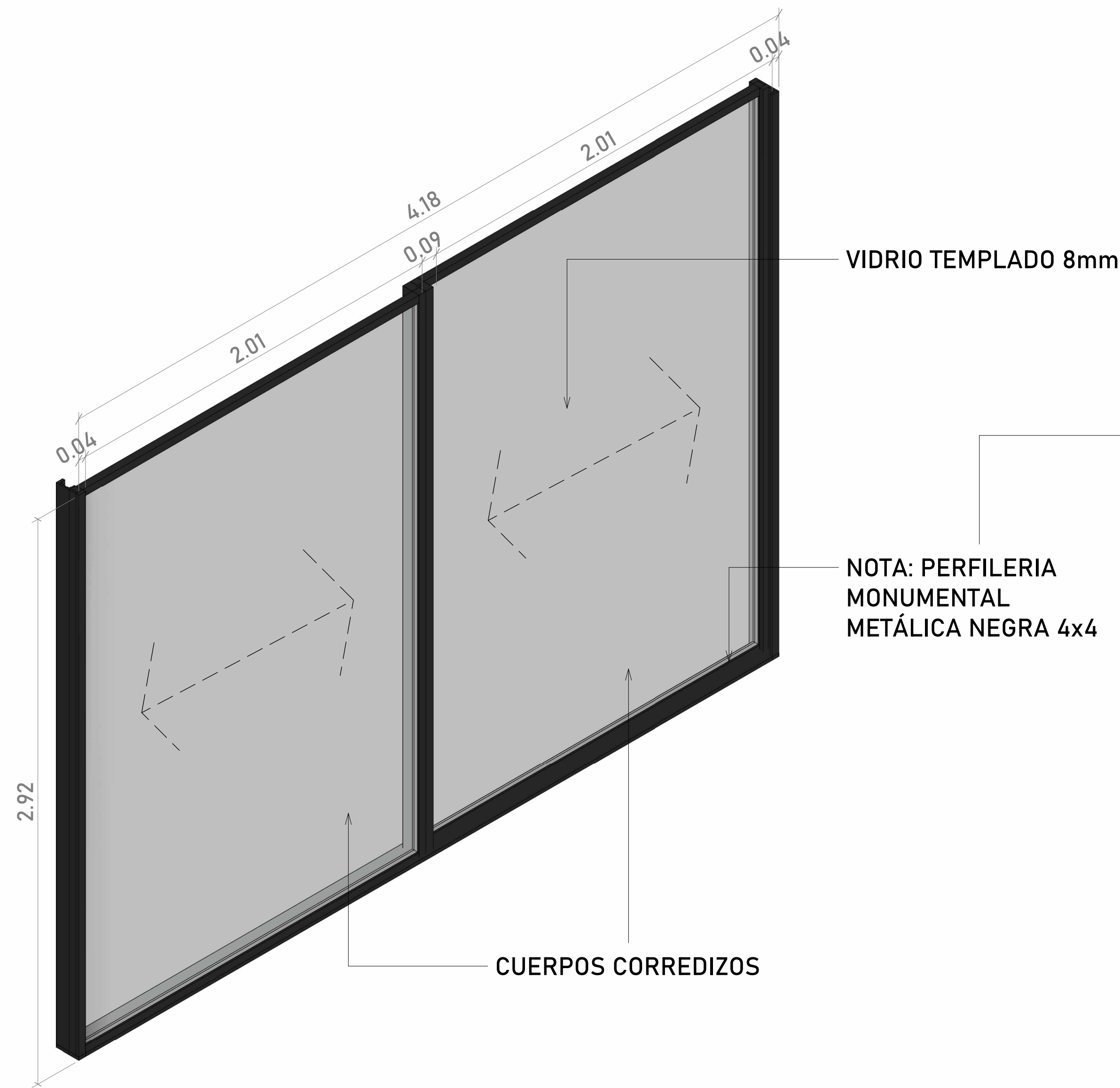
1 VENTANA CORREDIZA 1 HABITACIÓN PPAL 1: 25
