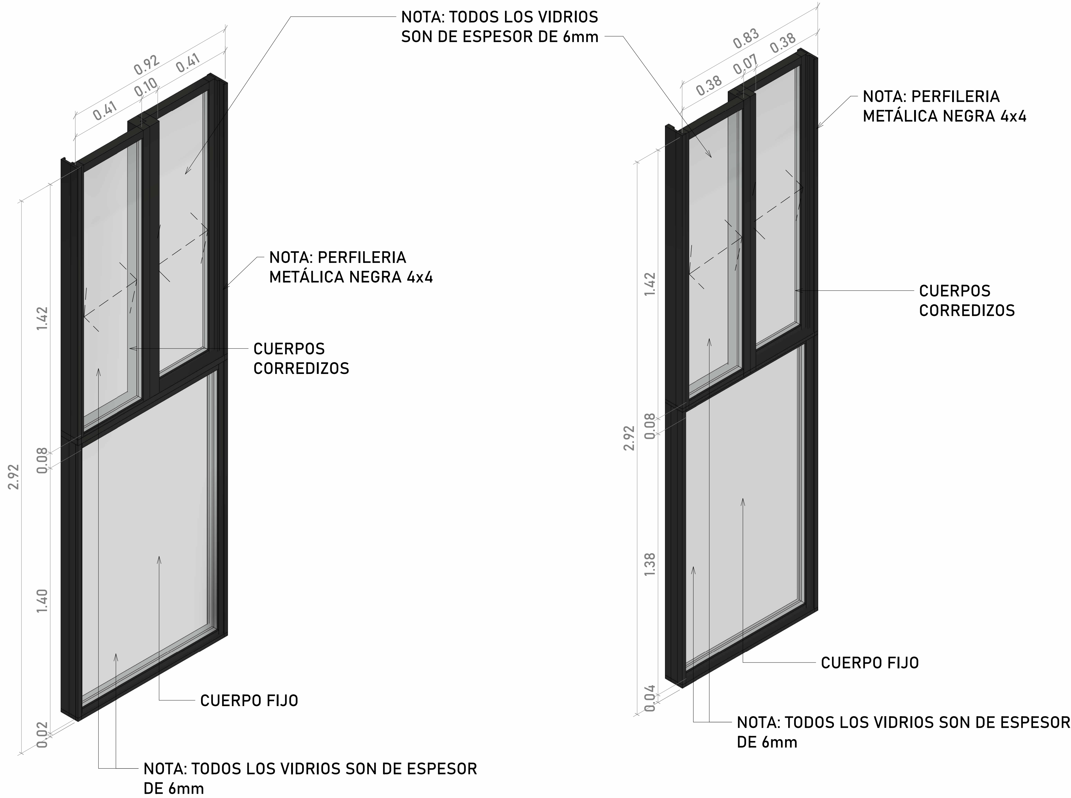
1 VENTANA 1 HAB SERVICIO 1: 10
