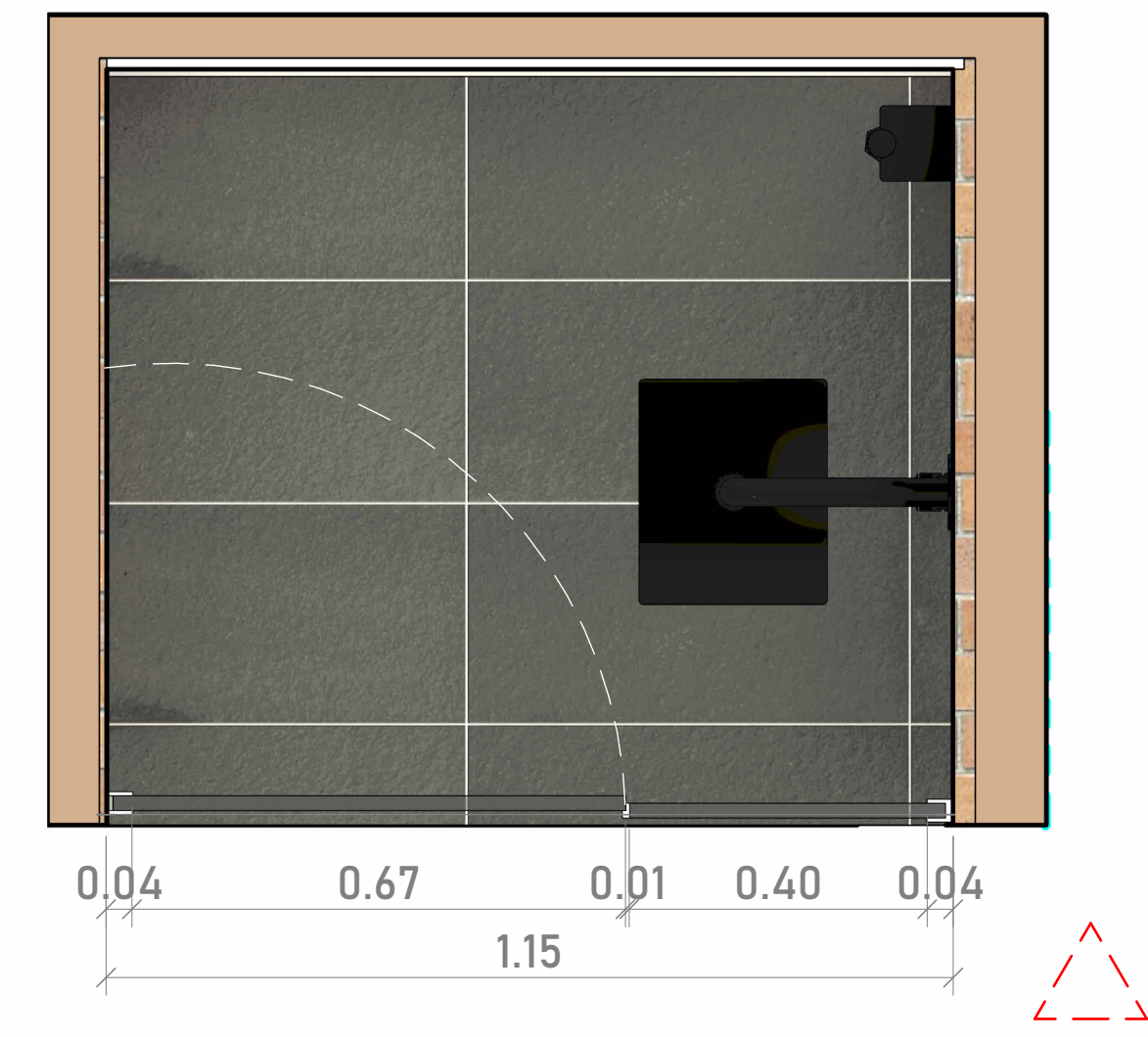
4 CABINA DUCHA HAB SERVICIO 1: 10
