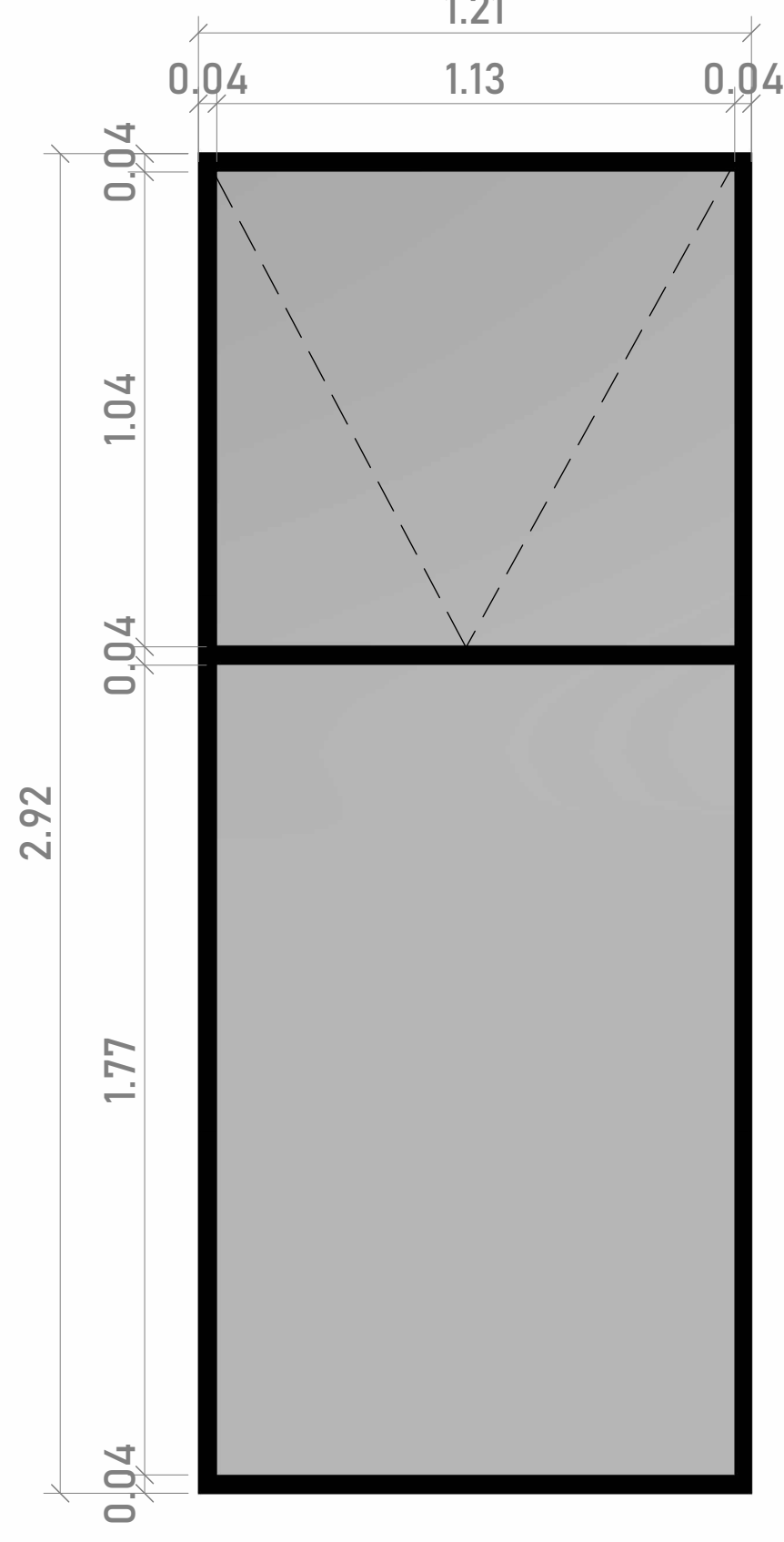
2 VENTANA DUCHA HABITACIÓN 2 1: 15
