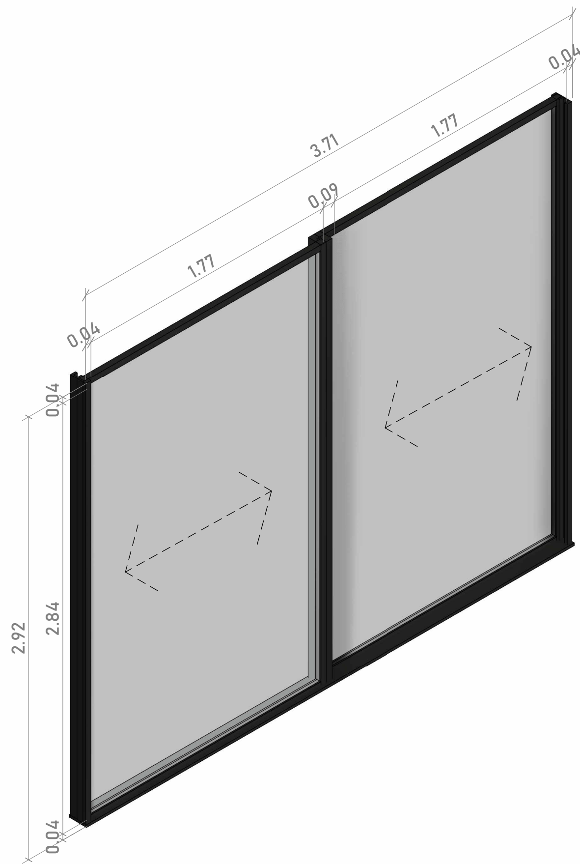
2 VISTA VENTANA CORREDIZA SALA TV 1: 20
