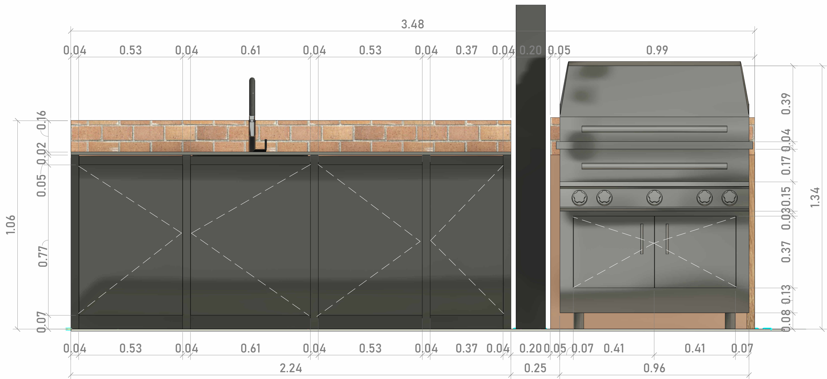
1 ALZADO MUEBLE BBQ EN METAL 1: 10
