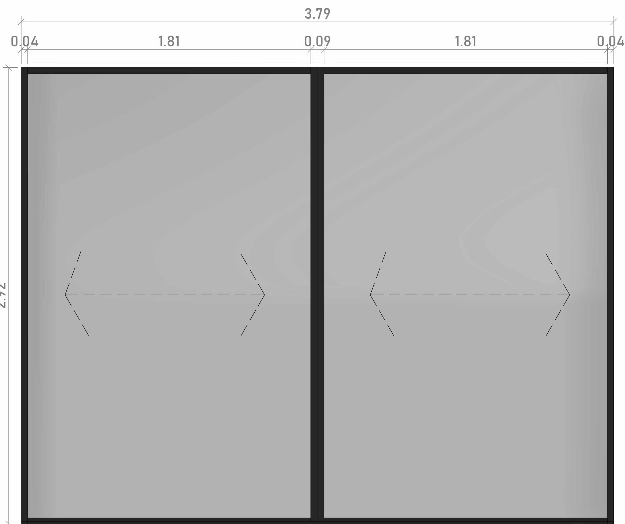
1 VENTANA CORREDIZA HABITACIÓN 3 1: 25
