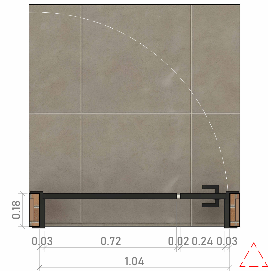
3 PUERTA METÁLICA HAB SERVICIO 1: 10
