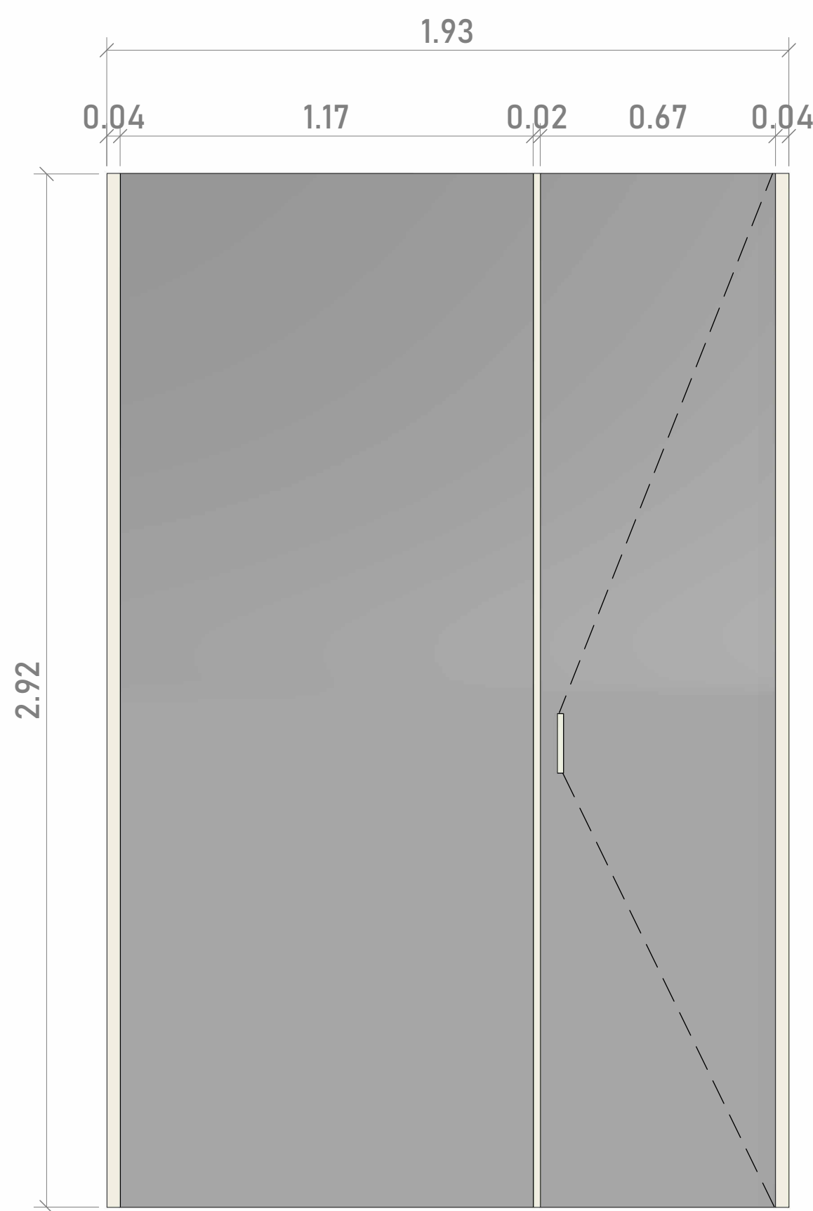
3 CABINA DUCHA HABITACIÓN 3 1: 25
