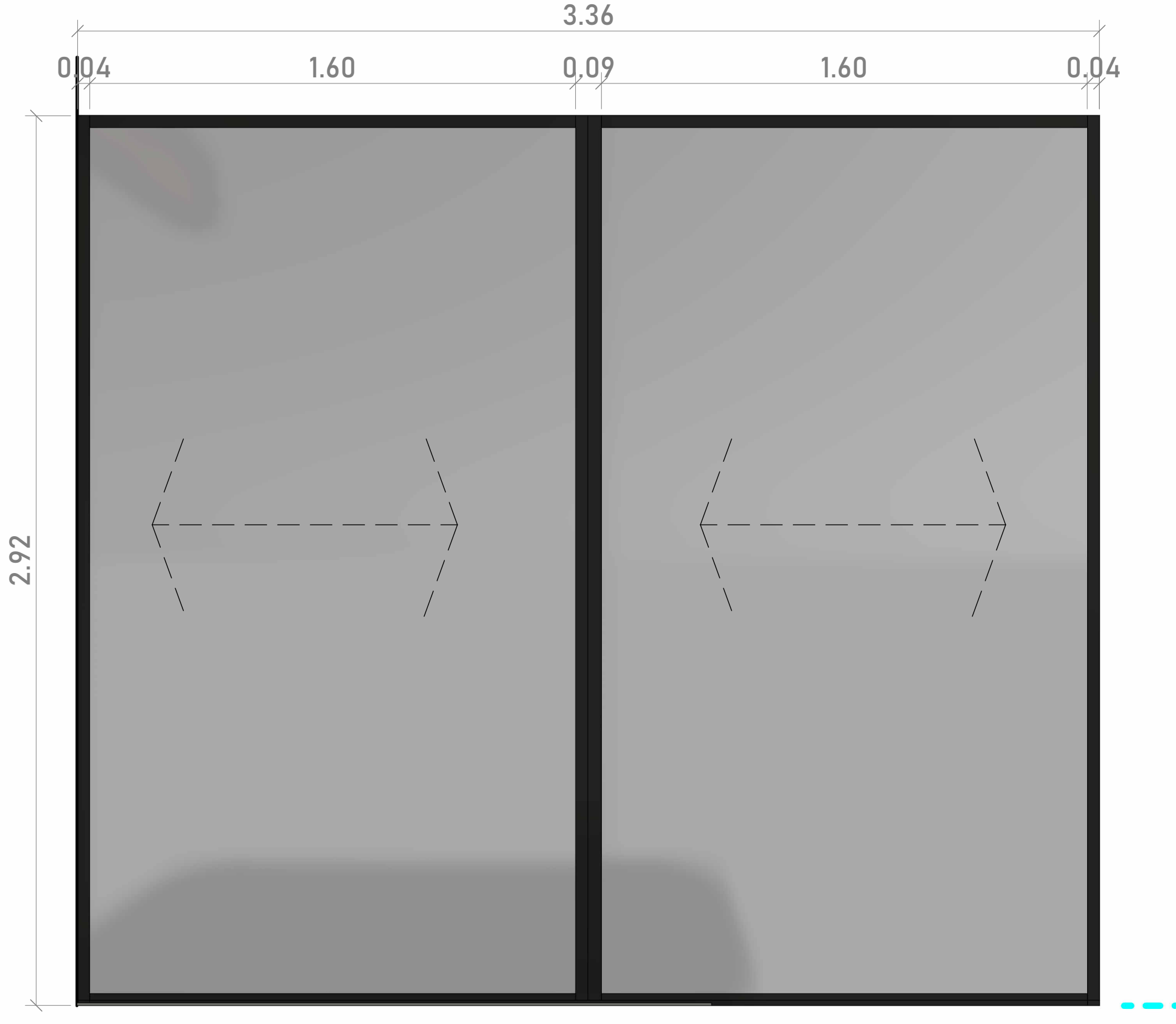
1 VENTANA CORREDIZA HABITACIÓN 2 1: 15
