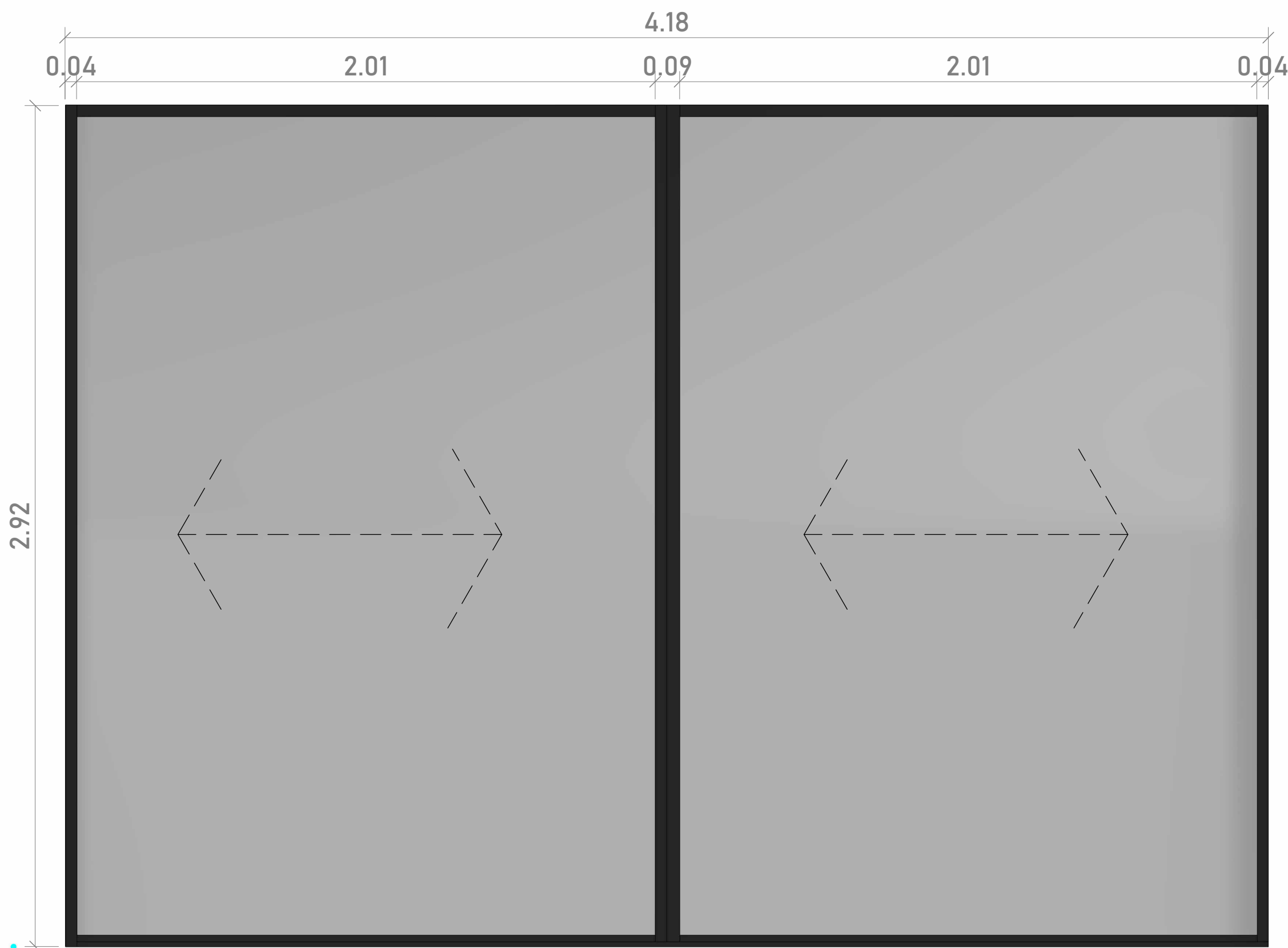
1 VENTANA CORREDIZA 1 HABITACIÓN PPAL 1: 25
