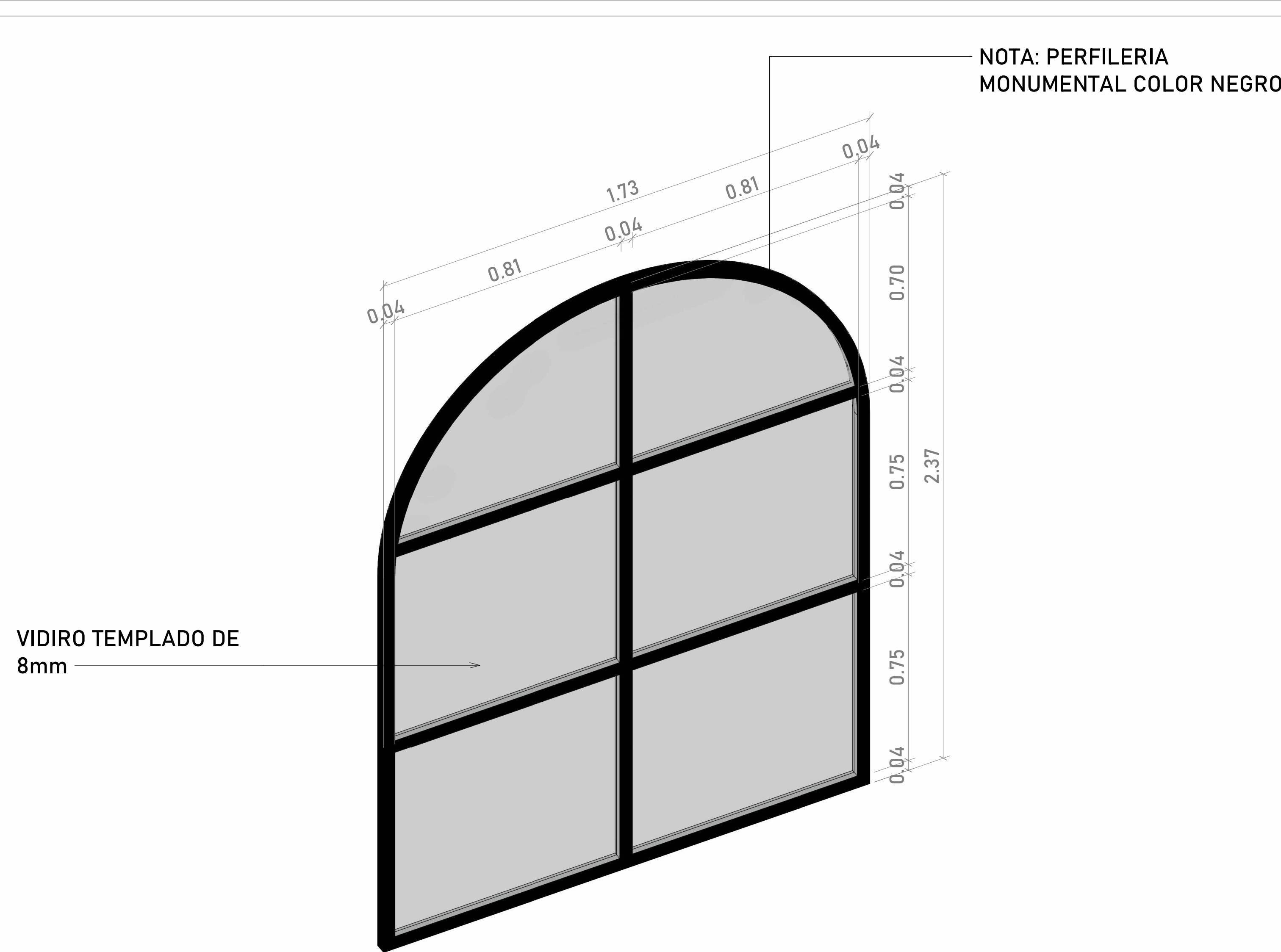
1 ISOMETRICO ARCO PERFILERIA METÁLICA 1: 10
