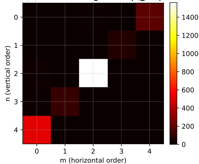
(b) Moment Magnitude |Q_{nm}|
