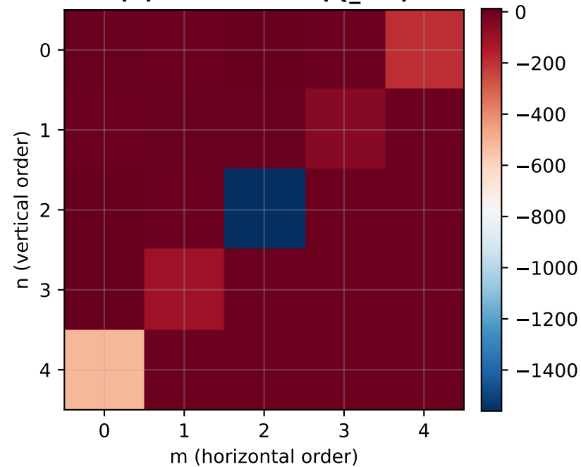
(d) Real Part \text{Re}(Q_{nm})
