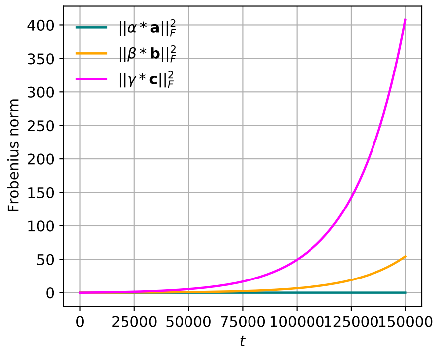
Norms vs t (eta=1.0)
