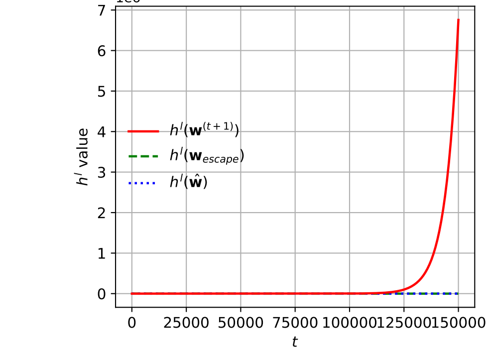
Lifted Loss vs t (eta=1.0)
