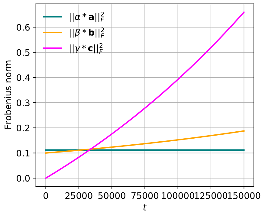
Norms vs t (eta=1.0)
