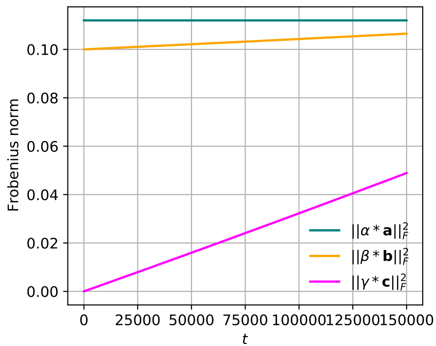
Norms vs t (eta=0.1)
