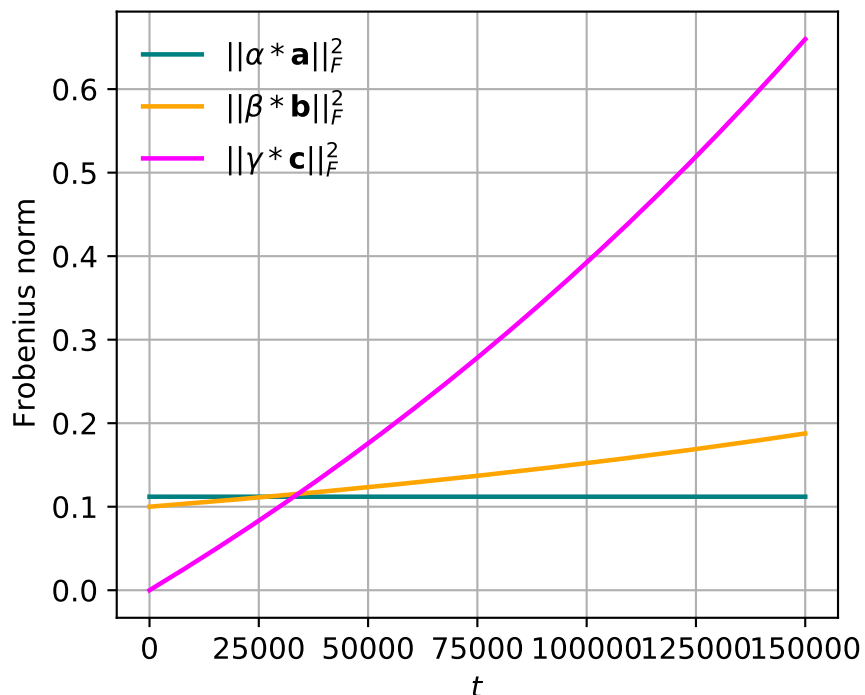
Norms vs t (rho=1.0)
