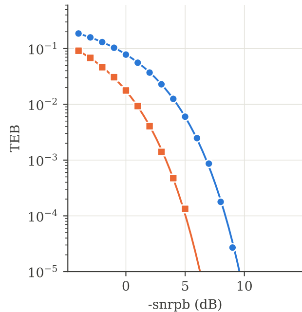
NRZ antipodal (-1, 1)
